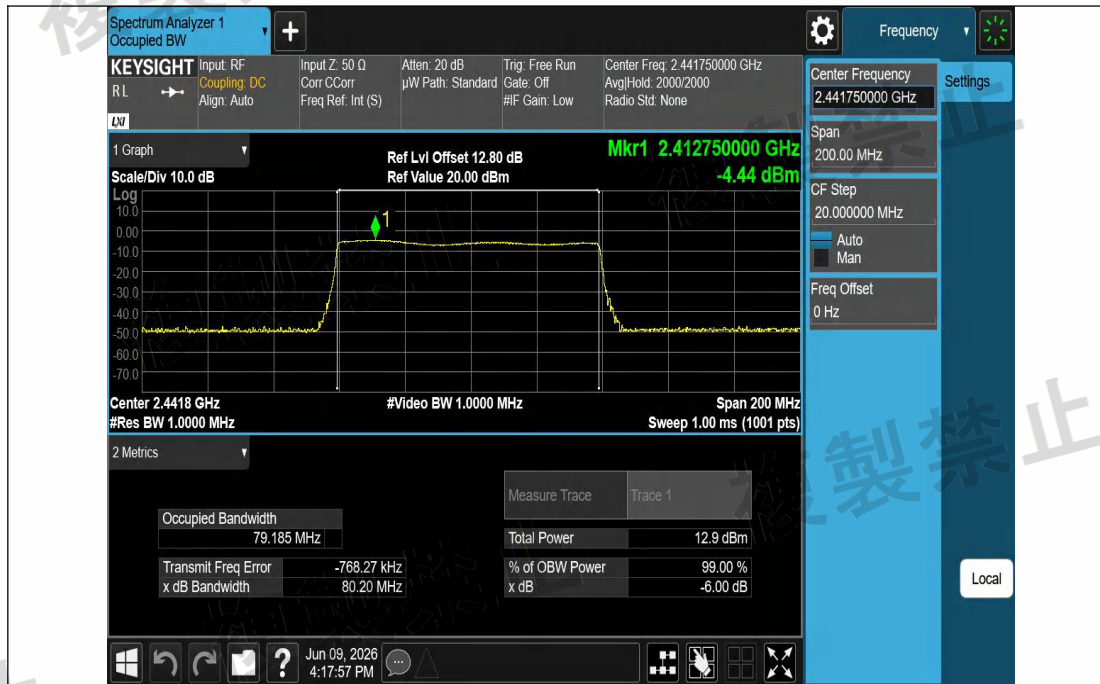
NTNV-2DH5-Ant1-Hop-PASS
