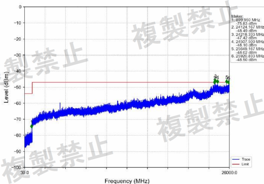
802.11n(HT20)_LCH_5180MHz_Ant1_NTNV
