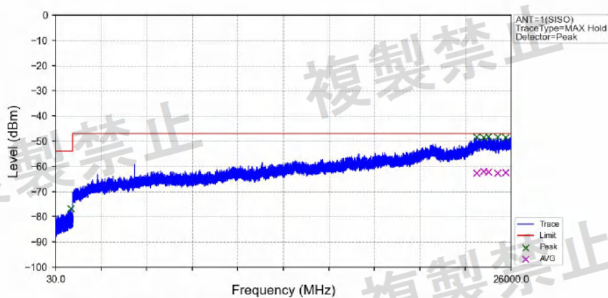
802.11ac(VHT40)_LCH_5270MHz_Ant1_NTNV
