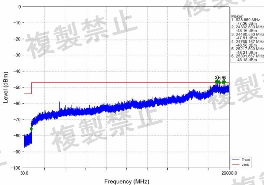
802.11n(HT40)_LCH_5270MHz_Ant1_NTNV
