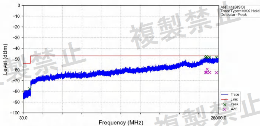
802.11a_MCH_5300MHz_Ant1_NTNV
