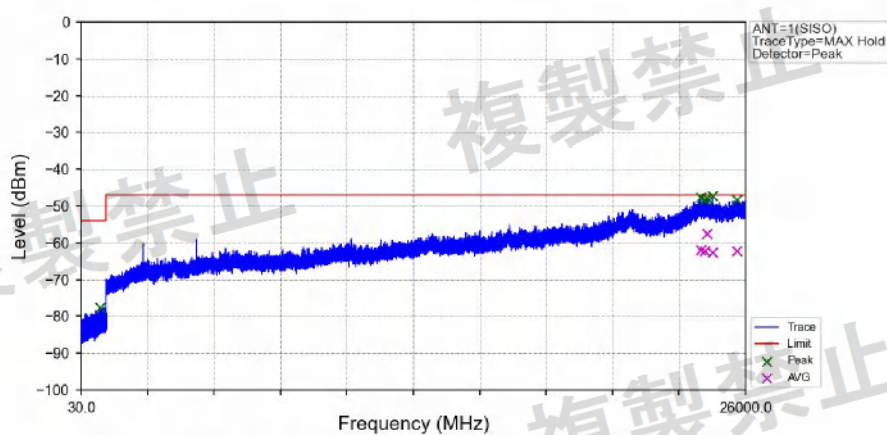
802.11a_LCH_5500MHz_Ant1_NTNV
