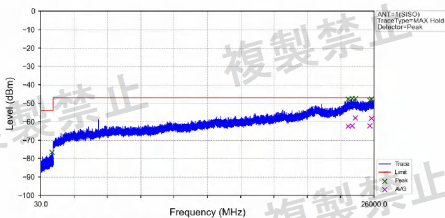
802.11ax(HEW40)_LCH_5270MHz_SU_ / _Ant1_NTNV
