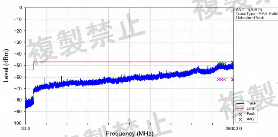
802.11ax(HEW20)_HCH_5700MHz_SU / _Ant1_NTNV
