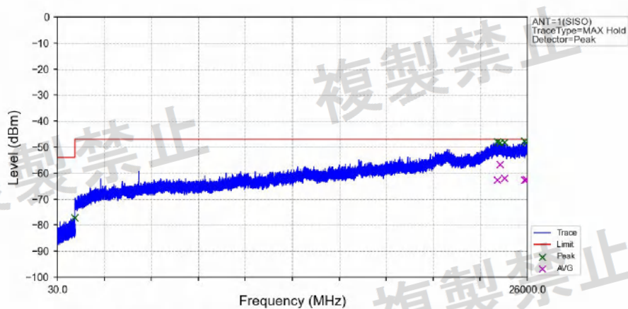
802.11n(HT20)_HCH_5320MHz_Ant1_NTNV
