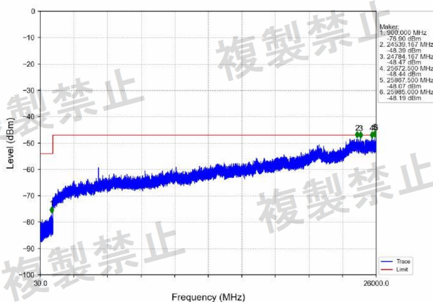
802.11n(HT20)_HCH_5700MHz_Ant1_NTNV
