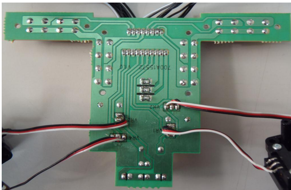
圖 6、設備 TX 印刷電路板銅軌面(廠牌: SANWA /型號: TX:AQUILA 6 ; RX:RX-71E)
