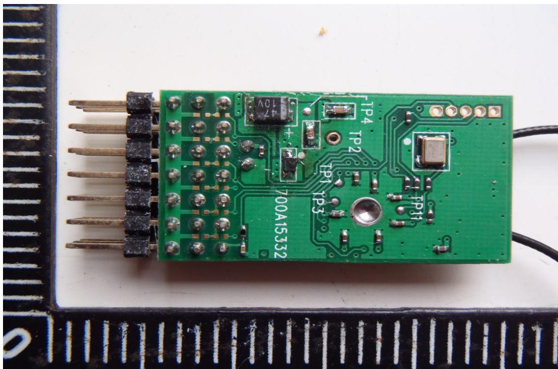
圖 20、設備 RX 印刷電路板銅軌面(廠牌: SANWA /型號: TX:AQUILA 6 ; RX:RX-71E)
