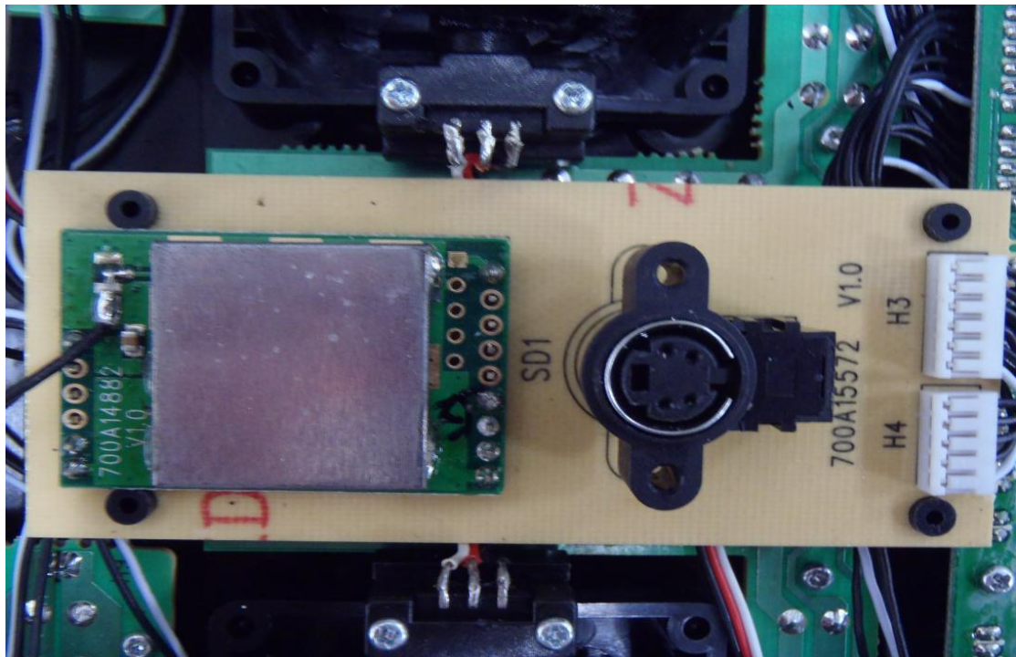
圖 14、設備 TX 印刷電路板銅軌面(廠牌: SANWA /型號: TX:AQUILA 6 ; RX:RX-71E)
