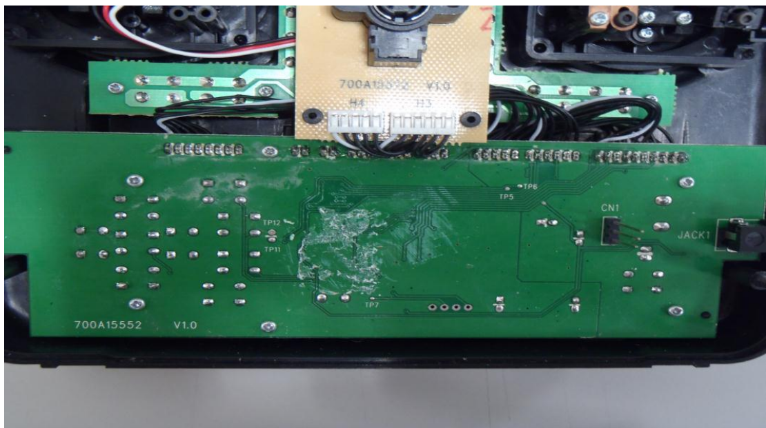
圖 12、設備 TX 印刷電路板銅軌面(廠牌: SANWA /型號: TX:AQUILA 6 ; RX:RX-71E)
