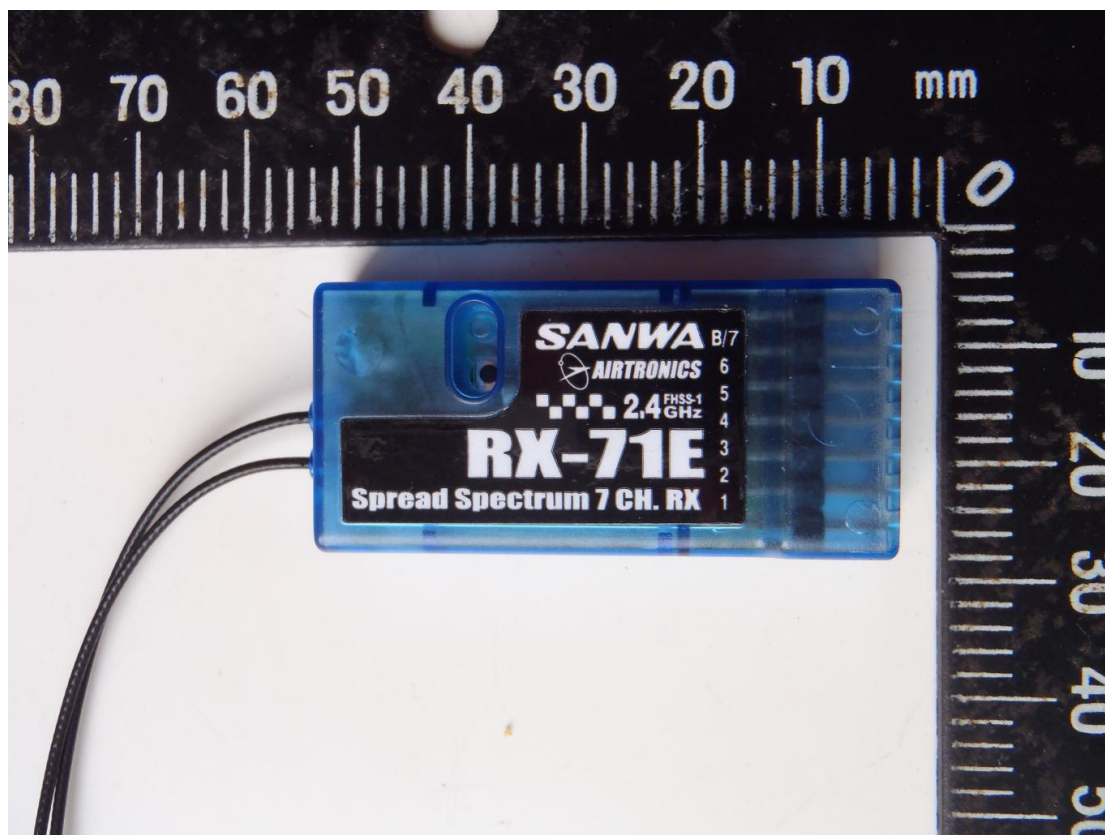
圖 16、設備 RX 背面照(廠牌: SANWA /型號: TX:AQUILA 6 ; RX:RX-71E)
