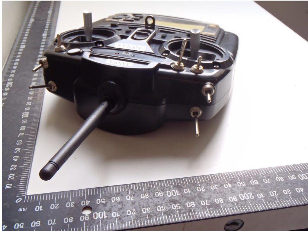
圖 4、設備 TX 側面(45 度角) (廠牌: SANWA /型號: TX:AQUILA 6 ; RX:RX-71E)
