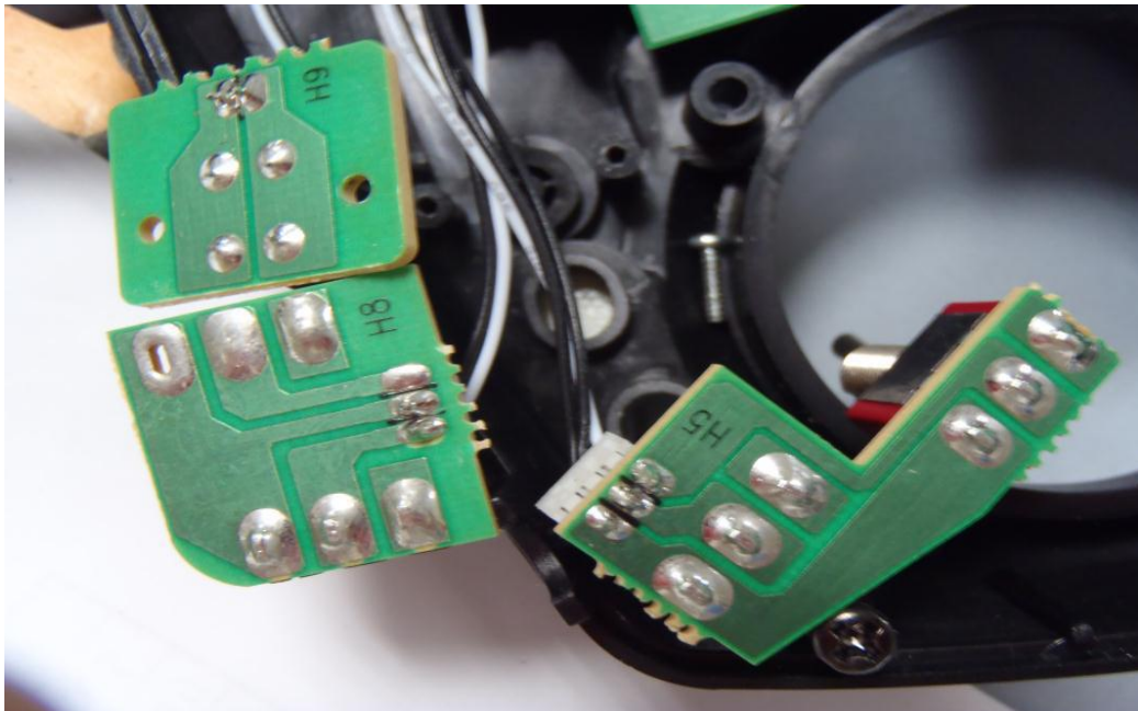
圖 8、設備 TX 印刷電路板銅軌面(廠牌: SANWA /型號: TX:AQUILA 6 ; RX:RX-71E)
