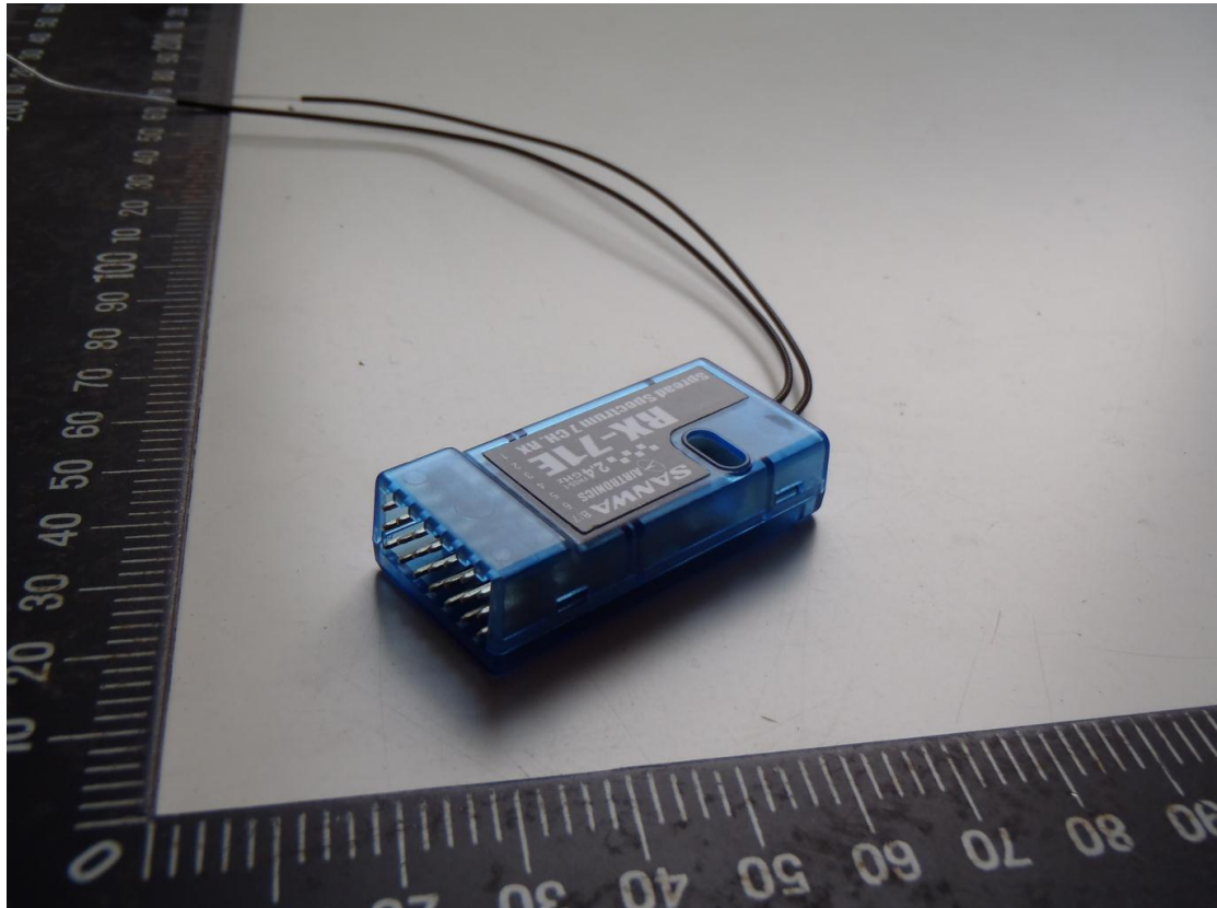
圖 18、設備 RX 側面照(廠牌: SANWA /型號: TX:AQUILA 6 ; RX:RX-71E)
