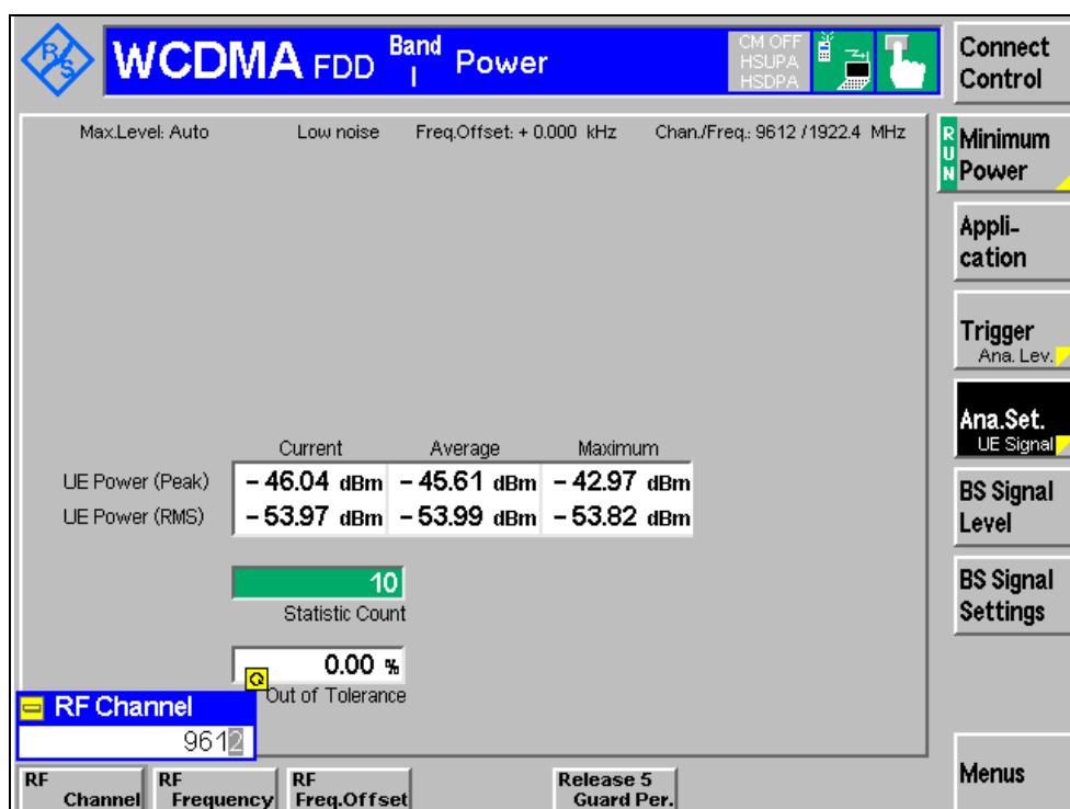
附件四之一：功率控制狀態下之最小平均輸出功率：測試頻道 9612 (1922.4 MHz)
