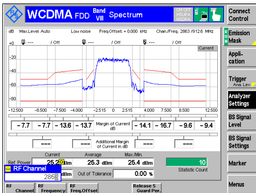
附件十三之三：發射頻譜波罩：測試頻道 2863 (912.6MHz)
