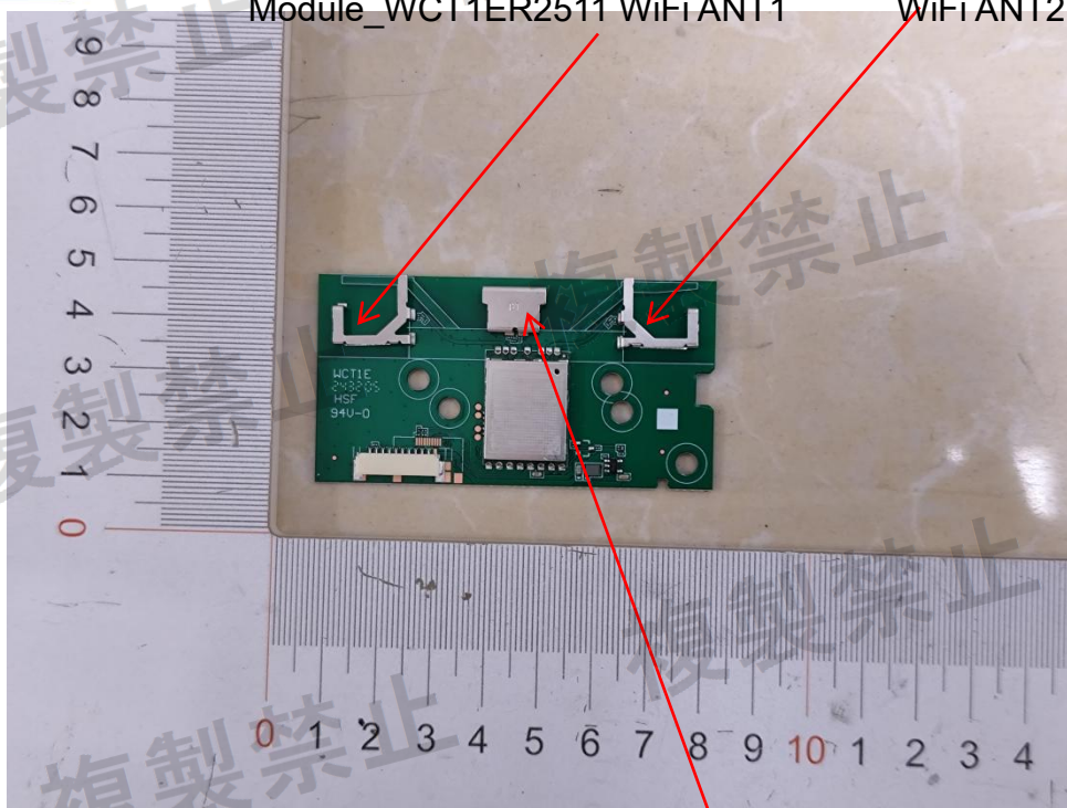
Module_WCT1ER2511 BT ANT
