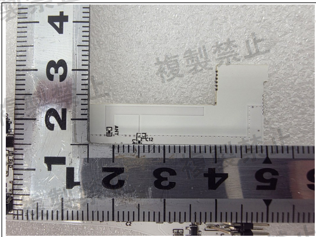
<BLE Antenna>
