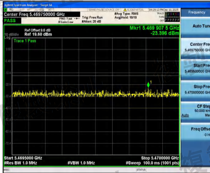
NTNV_11AX80SISO_Ant1_5530_5469.5~5470
