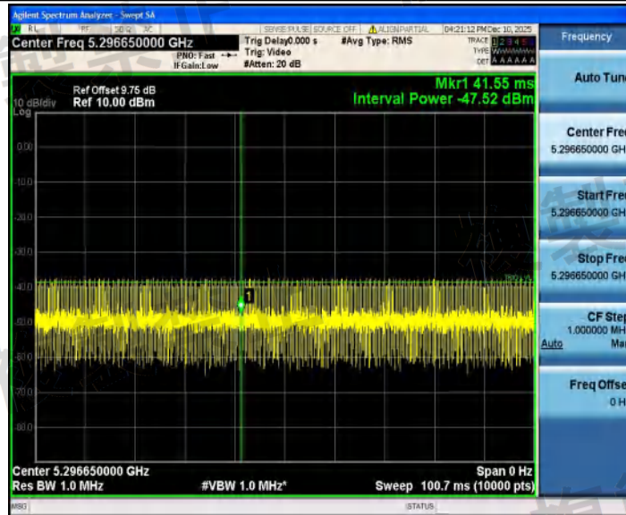
NTVN_11AX80SISO_Ant2_5210_5296.66_Ant2
