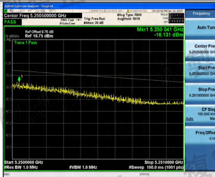
NTNV_11AX80SISO_Ant1_5210_5250~5251
