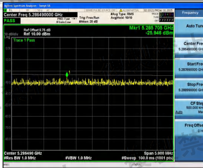
NTVN_11AC80SISO_Ant1_5210_5286.49_Ant1
