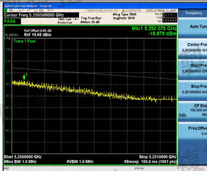
NTNV_11AX80SISO_Ant2_5210_5250~5251
