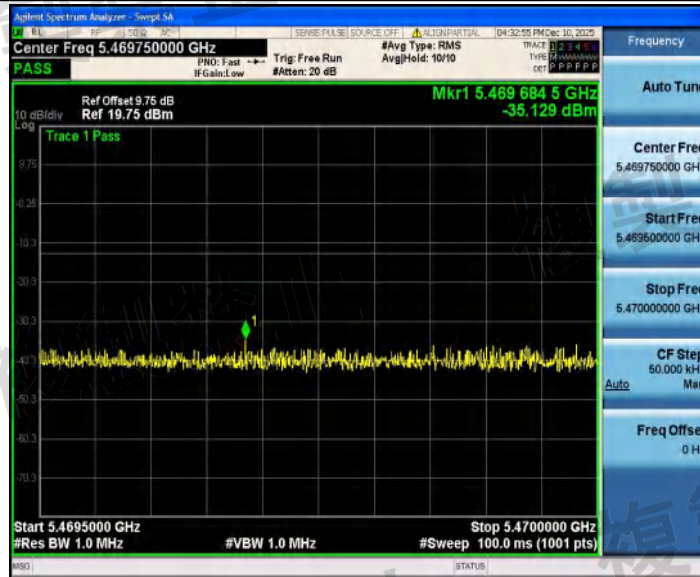
NTNV_11AX80SISO_Ant1_5610_5469.5~5470
