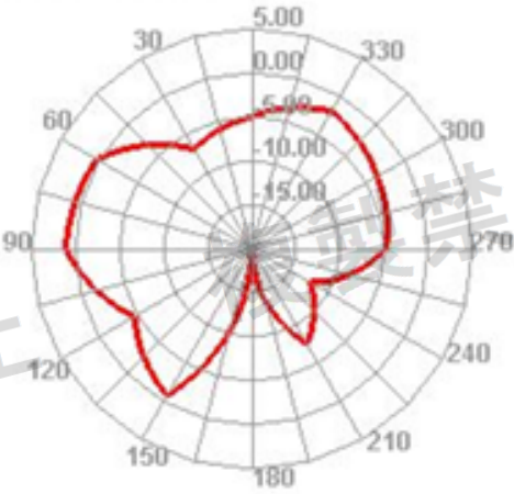
5150.000MHz E2
