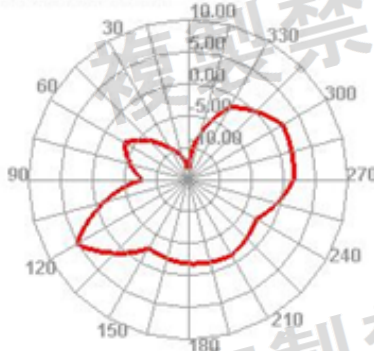
5850.000MHz E1
