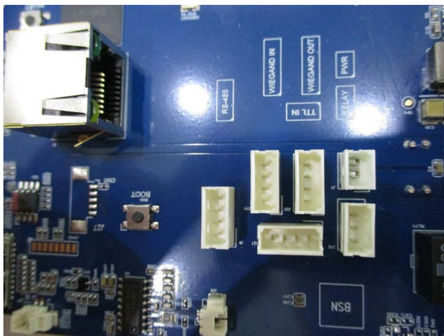
I/O Port 照 2
