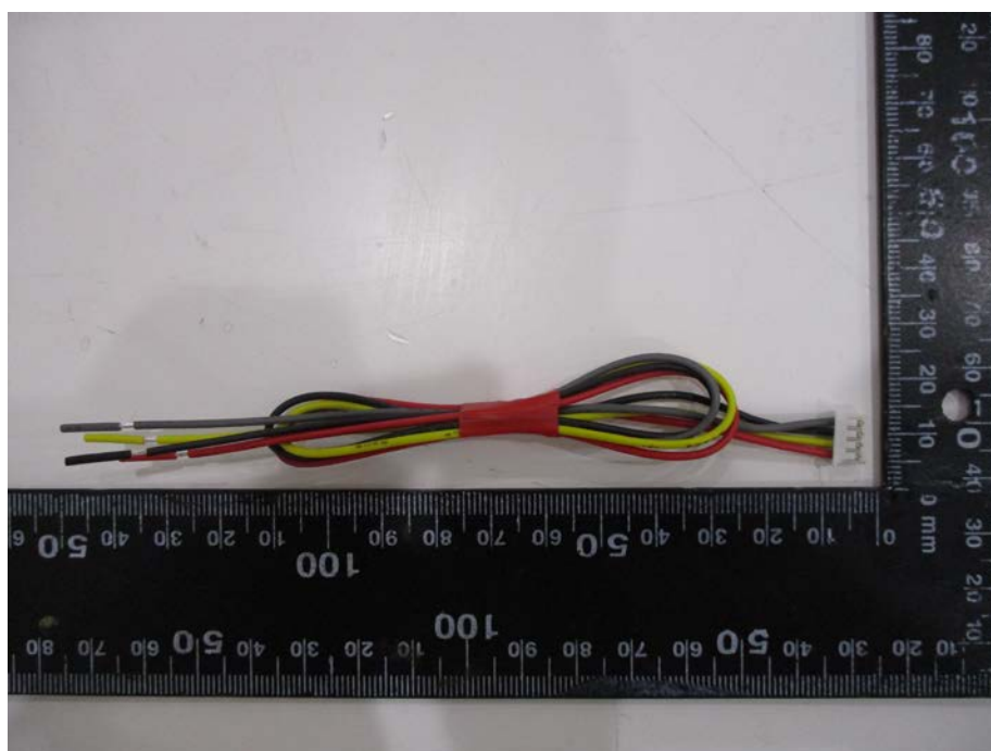
connection cable 4 pins(TTL)
