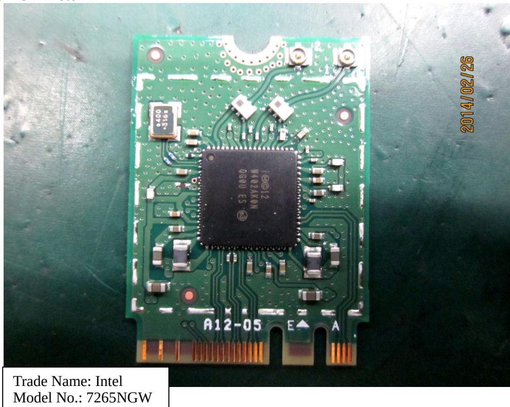
(10) EUT Photo
