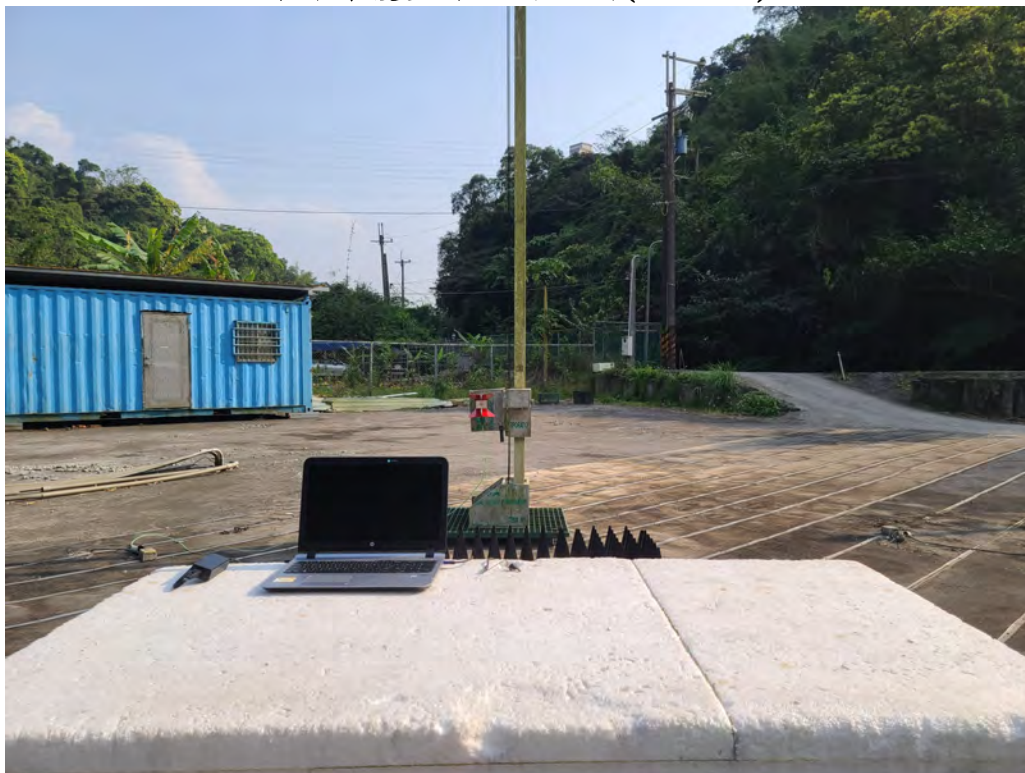
輻射干擾量測之配置照片(1 G 以上)
