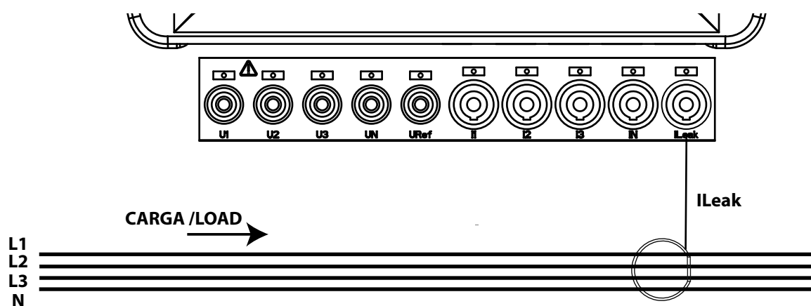
Figura 24: Podłączenie prądu upływowego, ILeak (MYeBOX 1500).
