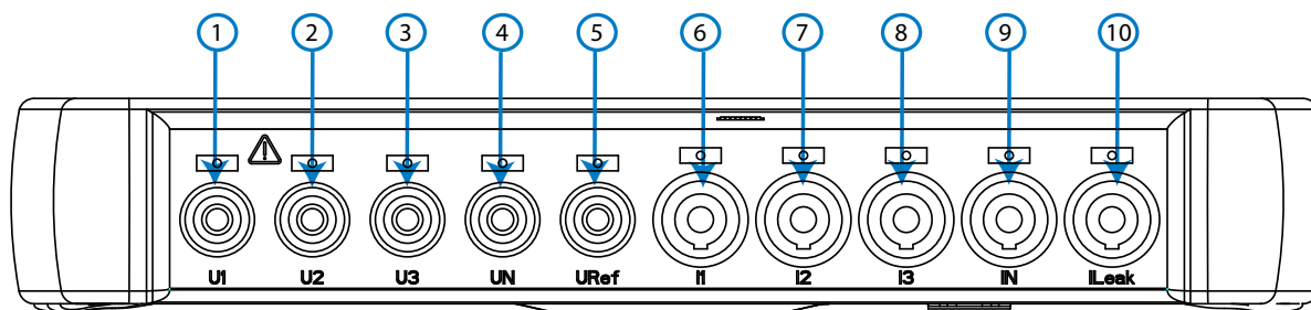
Figura 12:Zaciski MYeBOX 1500, część dolna.
