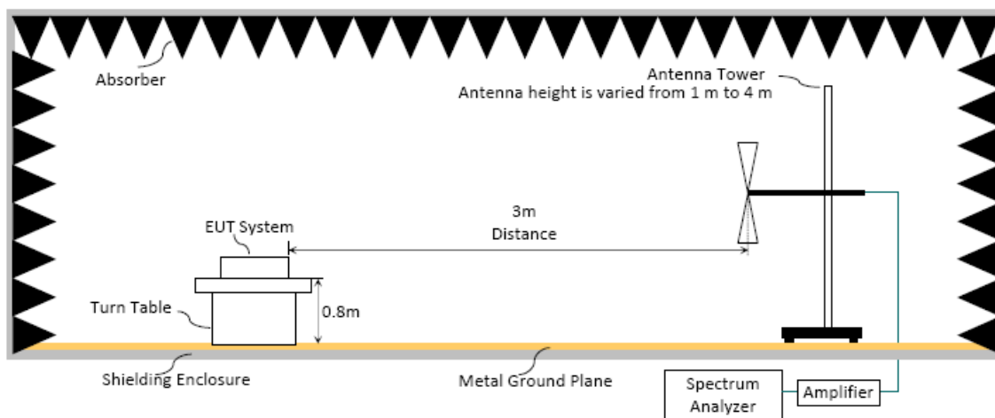
圖 2: 量測場地(Fully Anechoic Chamber)量測頻率高於 1GHz 之測試配置
