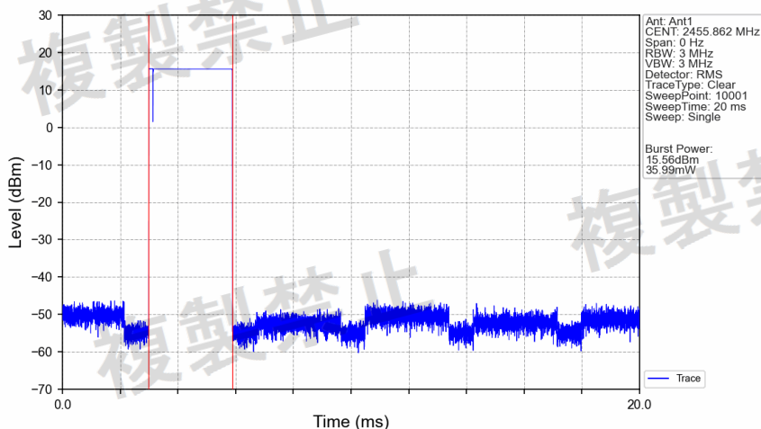
8DPSK_3DH5_HOPP20_Ant1_NTNV
