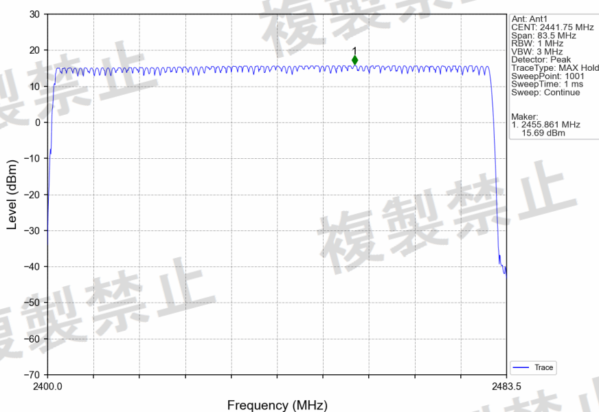
8DPSK_3DH5_HOPP20_Ant1_NTHV
