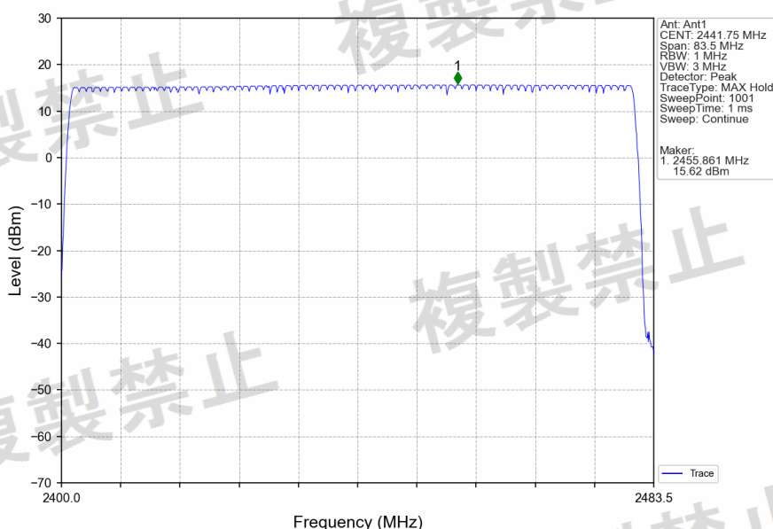
GFSK_DH5_HOPP20_Ant1_NTHV
