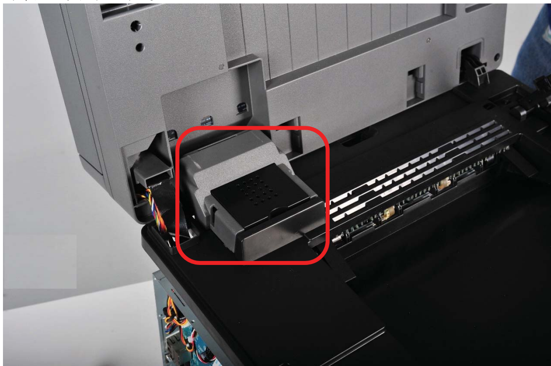
相片 6：特寫照，傳真模組(廠牌:Lexmark, 型號:LEX-M14-002), 位於照片中紅框所標示的掃描器平台下方的位置
