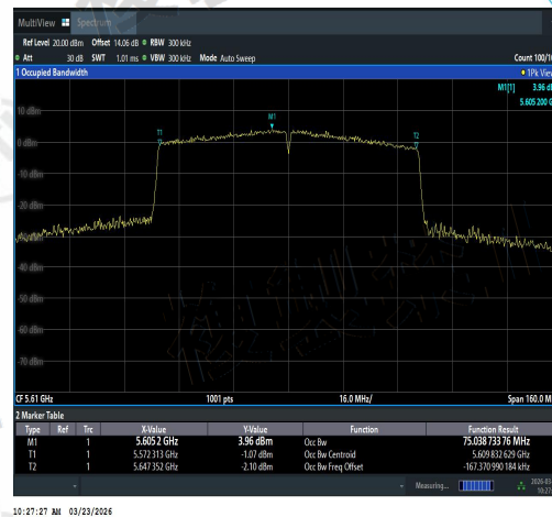
NTNV-11AC80SISO-Ant1-5610-PASS
