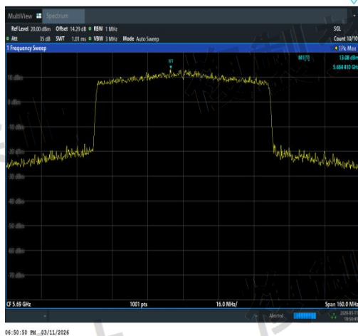
NTNV-11AX80SISO-Ant3-5690-TPC_H-PASS
