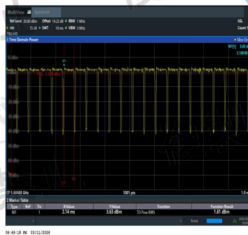
NTNV-11AX80SISO-Ant3-5610-TPC_H-PASS
