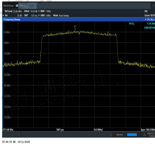
NTNV-11AX80SISO-Ant1-5690-TPC_H-PASS
