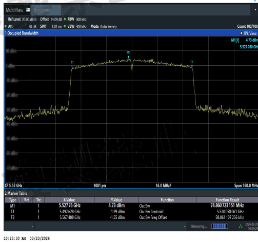
NTNV-11AC80SISO-Ant1-5530-PASS
