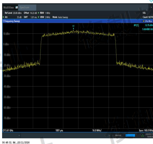
NTNV-11AX80SISO-Ant3-5610-TPC_H-PASS
