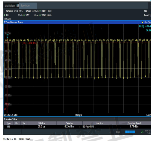
NTNV-11AX80SISO-Ant1-5530-TPC_H-PASS
