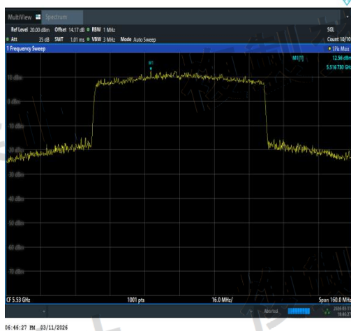
NTNV-11AX80SISO-Ant3-5530-TPC_H-PASS
