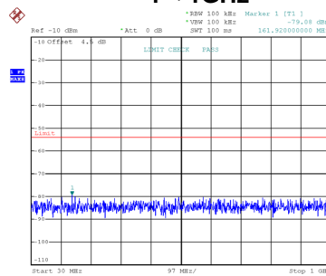
CH45 f < 1GHz
