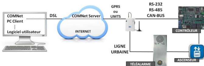
Figure F: exemple de système COMNet avec GSM500 GD NET utilisé comme passerelle pour la téléalarme
