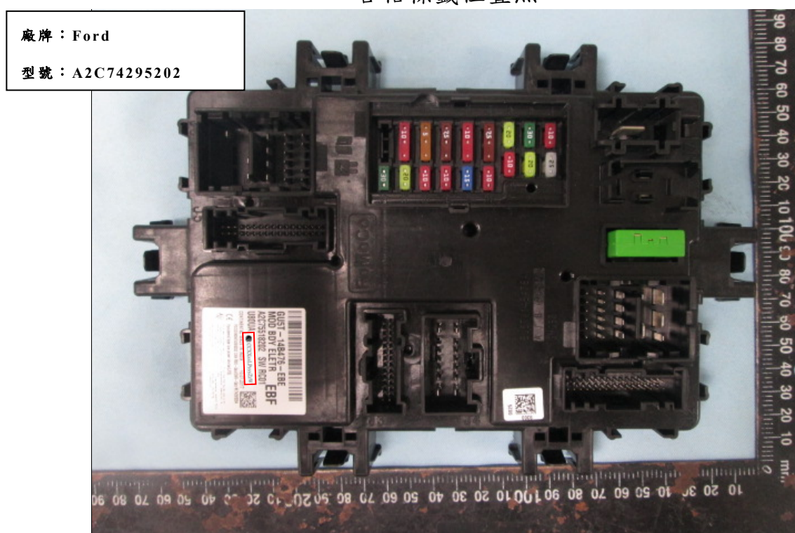
合格標籤位置照
