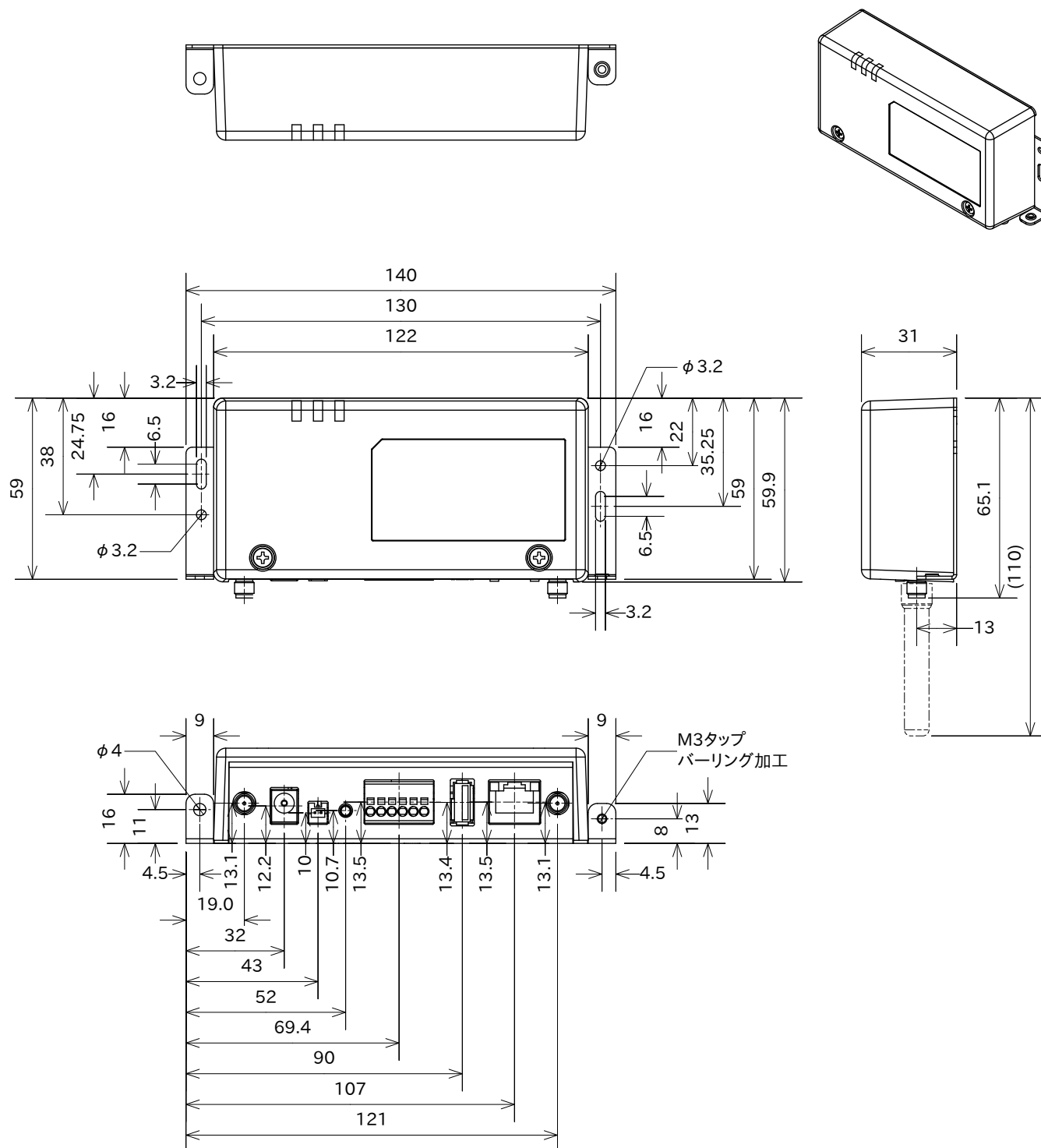
図 18.1 筐体形状図
