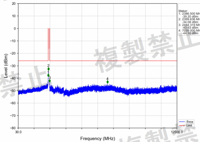
802.11n(HT40)_2422MHz_Ant1 (SISO)_NTNV
