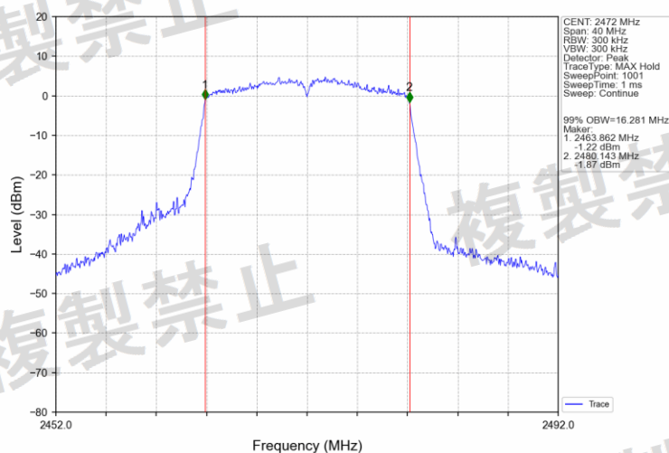
802.11g_2472MHz_Ant1 (SISO)_NTNV
