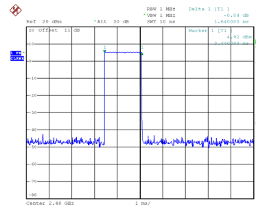
CH78-3DH3
