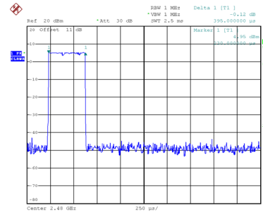
CH78-3DH1
