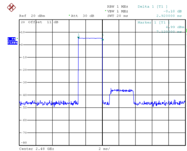
CH78-3DH5
