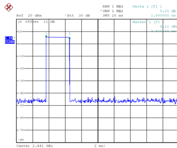
CH39-3DH5
