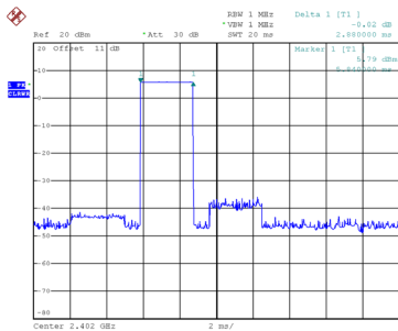
CH00-DH5
