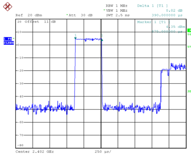
CH00-3DH1
