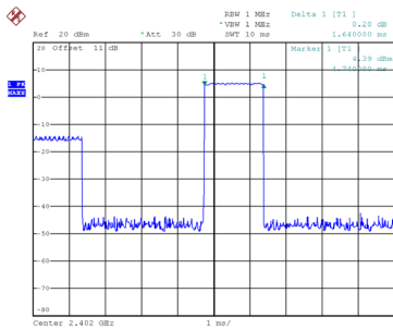
CH00-3DH3
