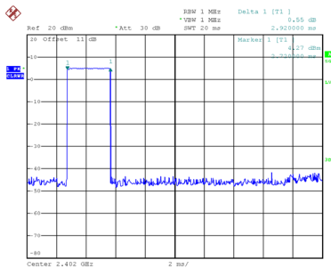
CH00-3DH5
