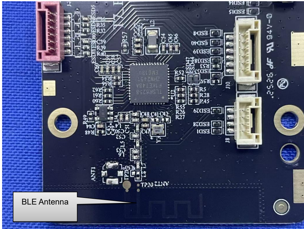
BLE Antenna Position
