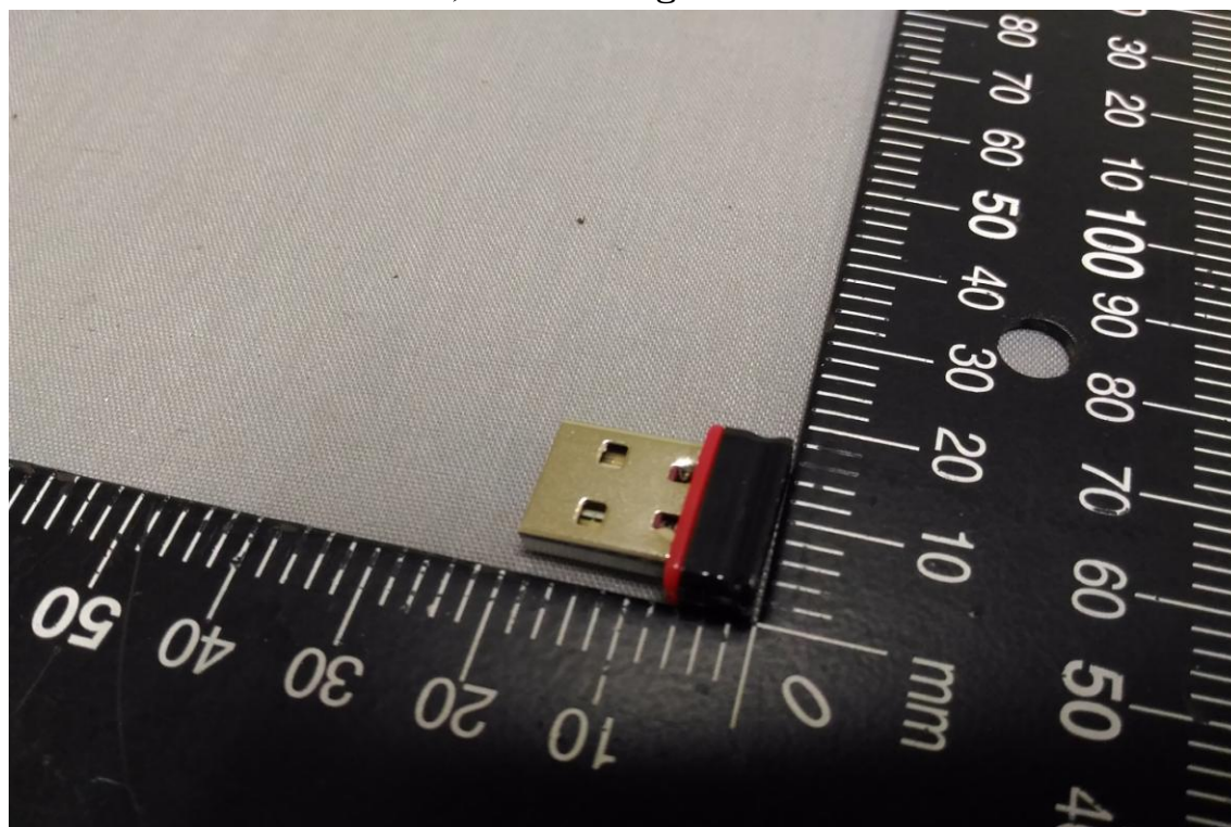
16) USB Dongle反面照
