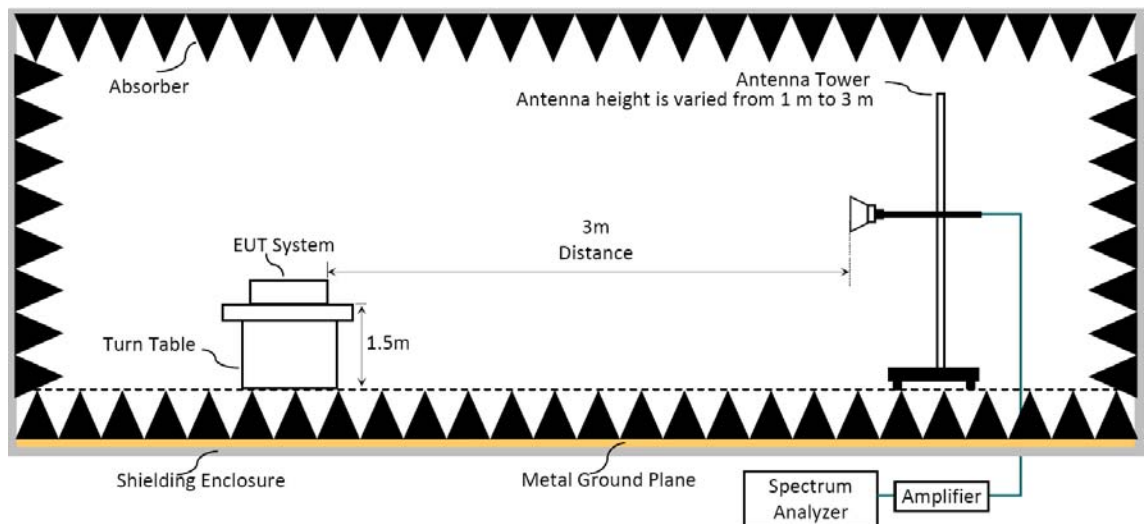
圖 2: 量測頻率高於 1GHz 之測試配置 Fully Anechoic Chamber
