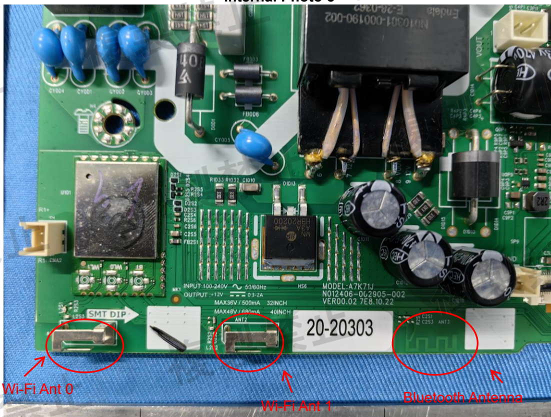
Antenna
