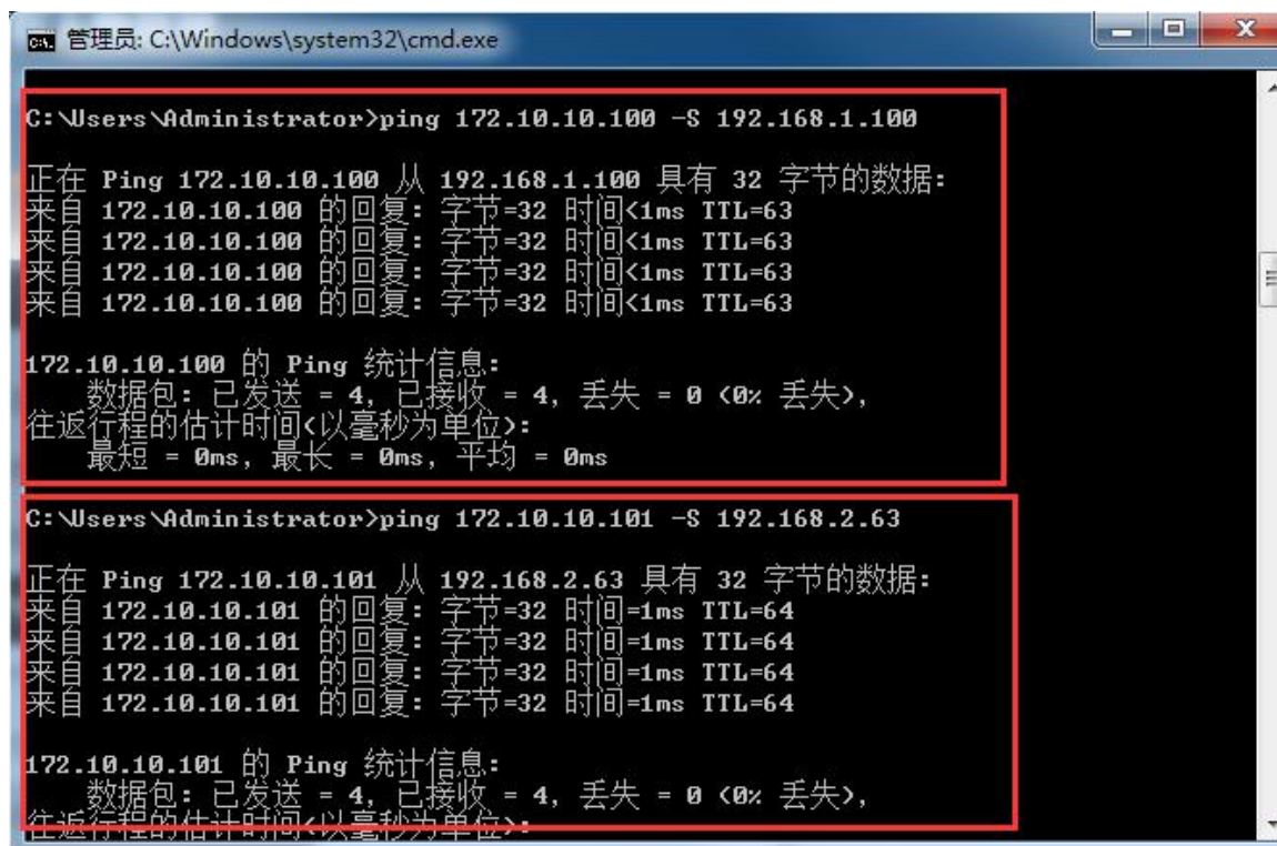
图 51 PPTP 搭建示例：网络互通
