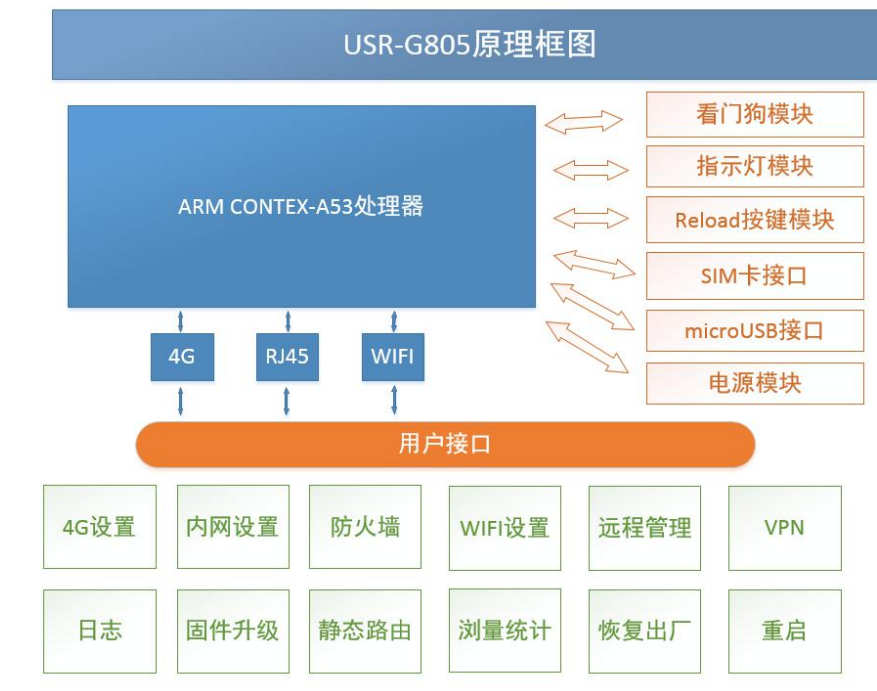
图 3 功能框图
