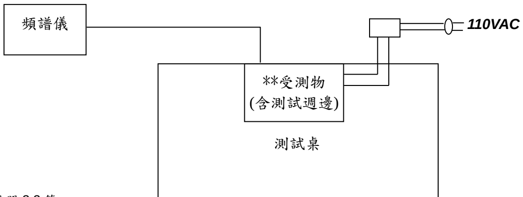
傳導量測配置圖
