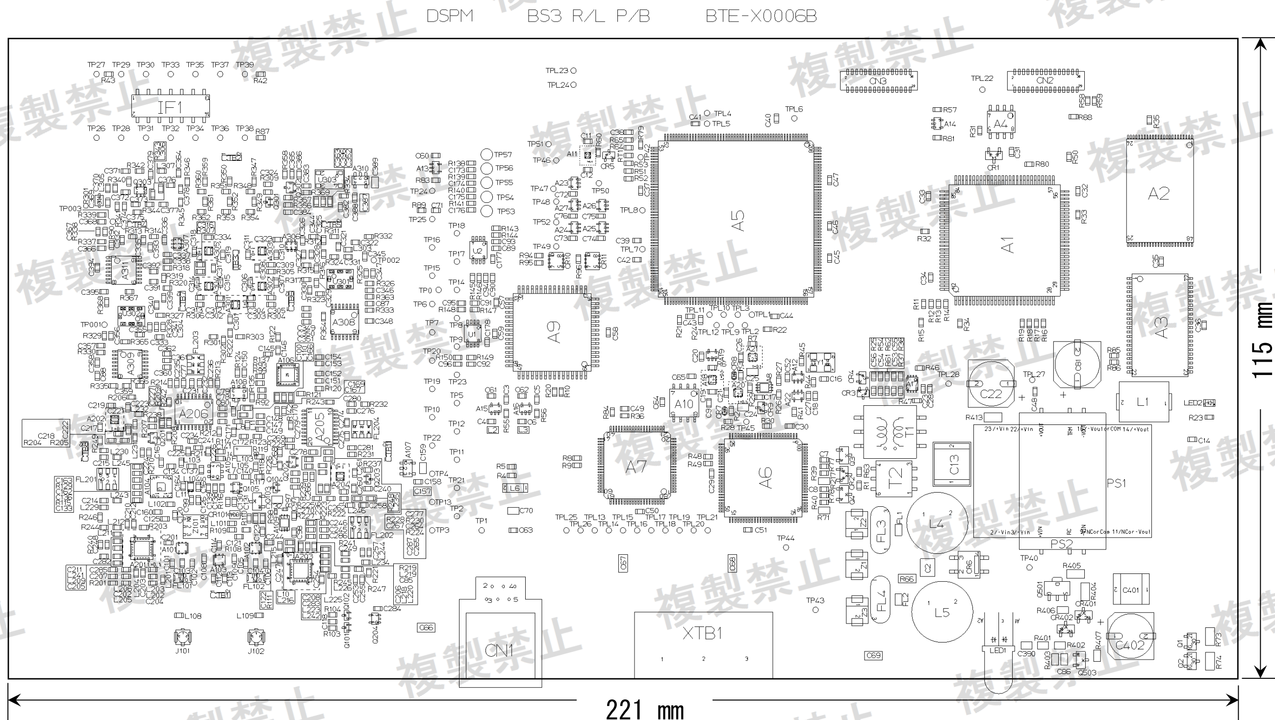
HL7-B500E0 本体基板 (BTE-X0006B) 部品配置図 (A 面)
