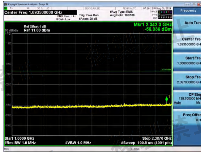
NTNV-11G-Ant1-2472-1000~2387-PASS
