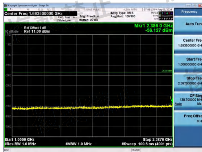
NTNV-11G-Ant1-2412-1000~2387-PASS
