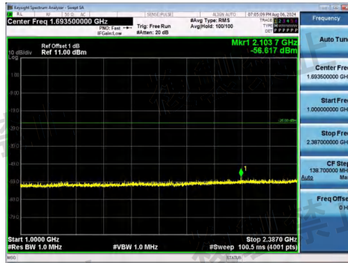
NTNV-11B-Ant1-2472-1000~2387-PASS
