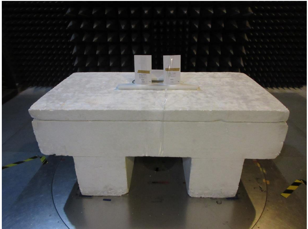
Radio1 Ant.21+23
