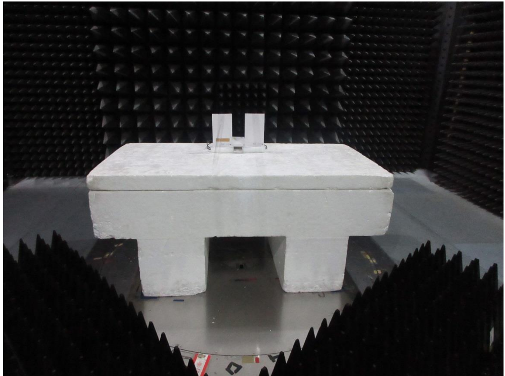
Radio1 Ant.21+23
