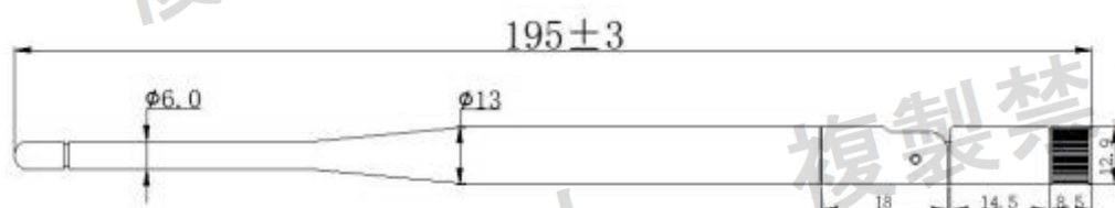
SMA-公头母针
