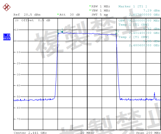
GFSK
