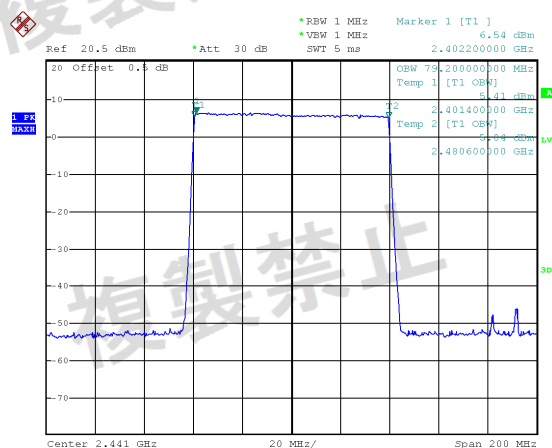
\pi/4 DQPSK
