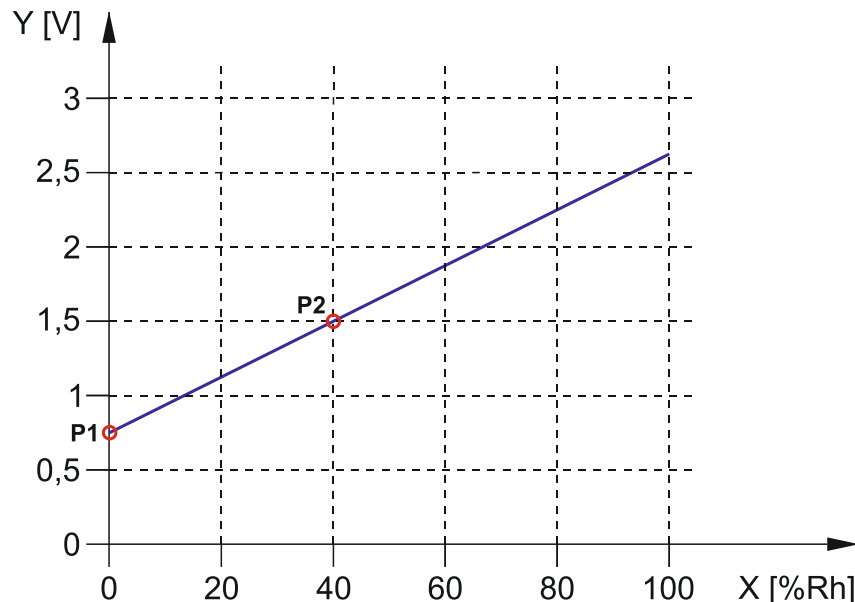
Abb. 22. Beispiel für lineare Kennlinie des Luftfeuchtesensors.
