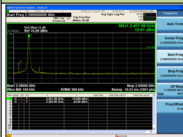
CH00 (2402MHz) LE(1Mbps)
