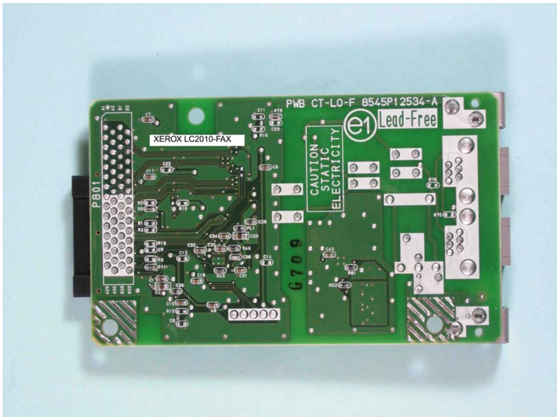
廠牌:XEROX 型號:LC2010-FAX 電路板
