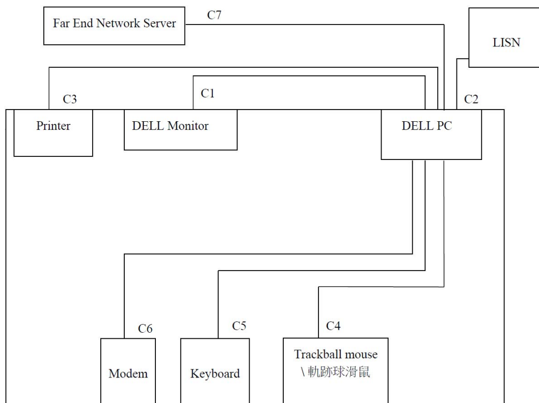
圖(一)電源傳導測試系統組成示意圖
