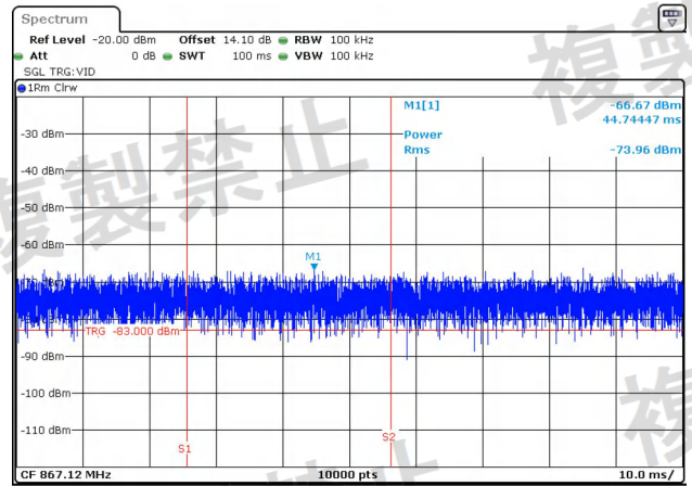
NTNV-11AC40-Ant2-5270-30~1000-PASS
