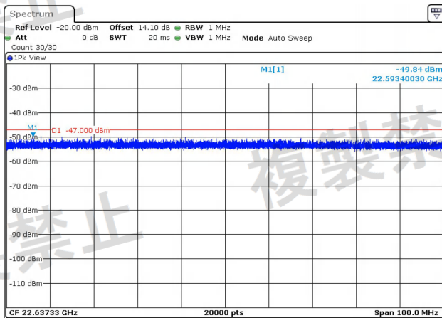
NTNV-11AC40-Ant1-5270-1000~26000-PASS
