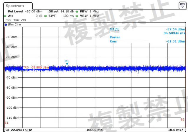
NTNV-11AC40-Ant1-5270-1000~26000-PASS
