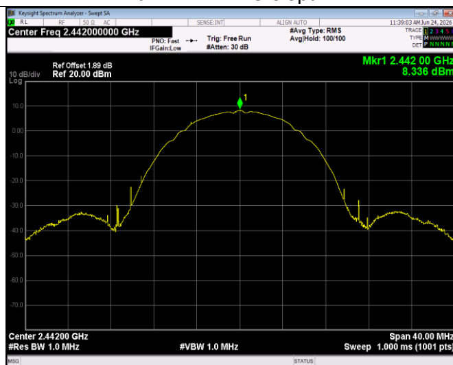
b 2442MHz
