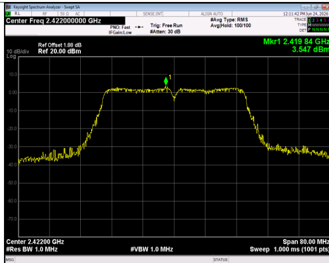
n40 2422MHz
