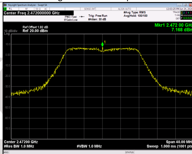
g 2472MHz
