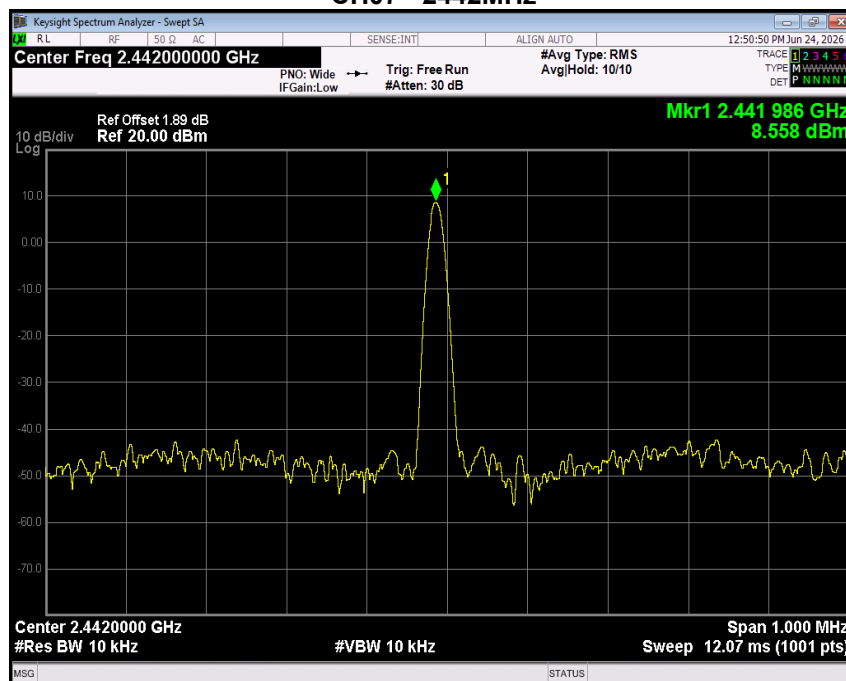
CH07 - 2442MHz
