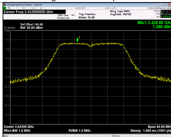
g 2442MHz
