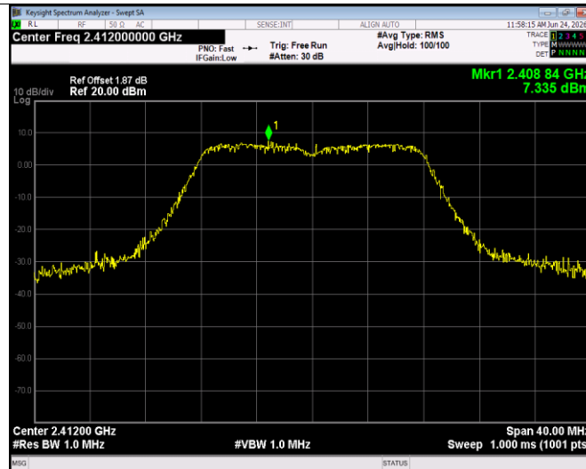
g 2412MHz
