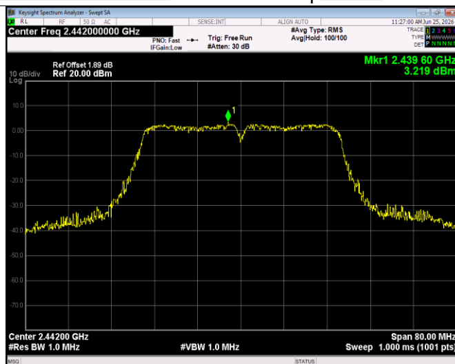
n40 2442MHz
