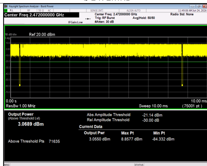
b 2472MHz
