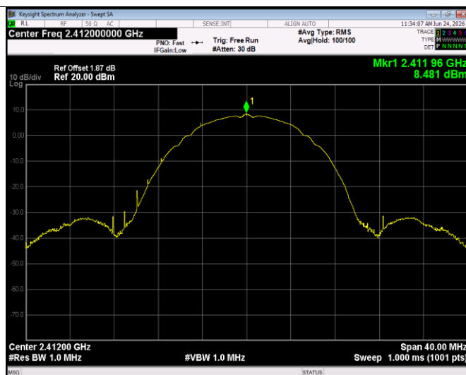
b 2412MHz
