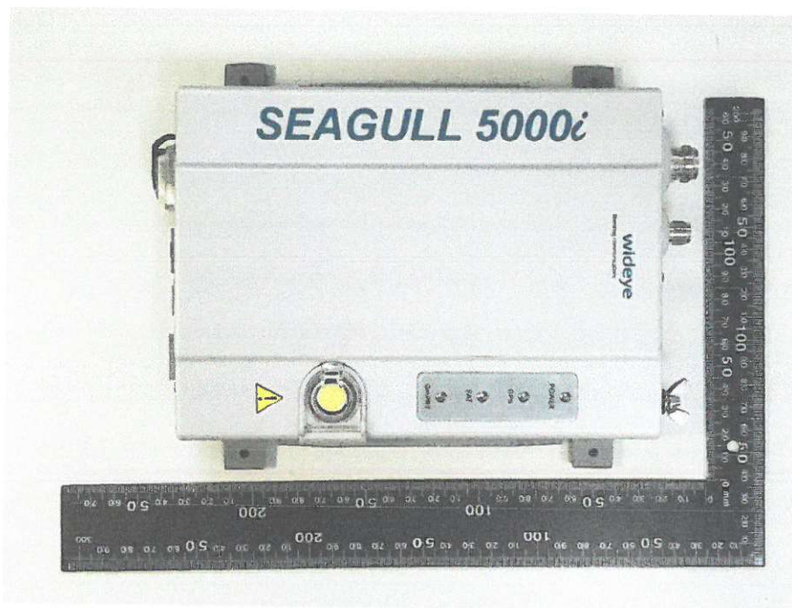
照片一：主機正面
