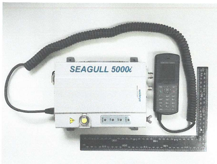
照片十二：主機與 Handset
