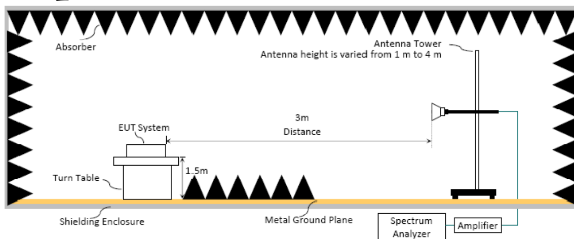
圖 2: 量測場地(3m Semi Anechoic Chamber)量測頻率高於 1GHz 之測試配置
