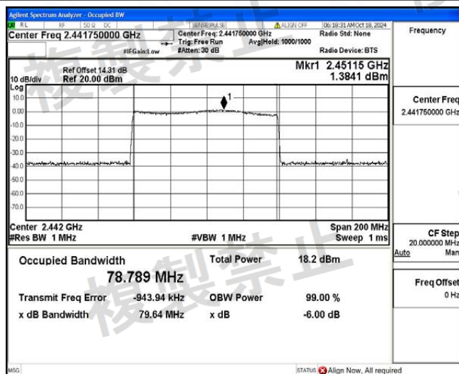
NTLV_3DH5_Ant1_Hop
