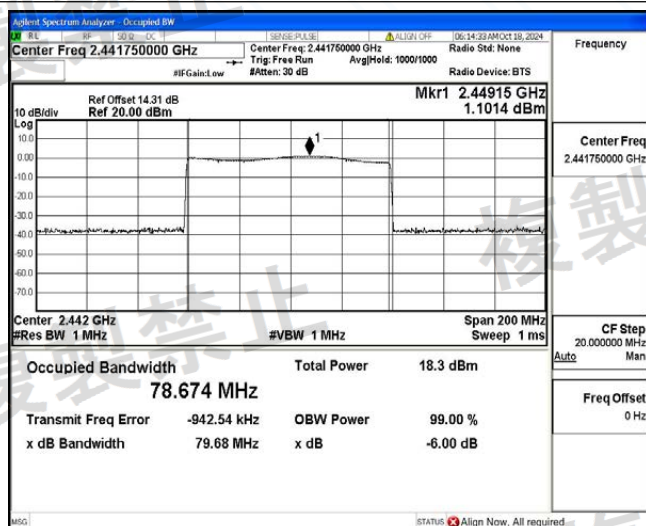
NTHV_2DH5_Ant1_Hop
