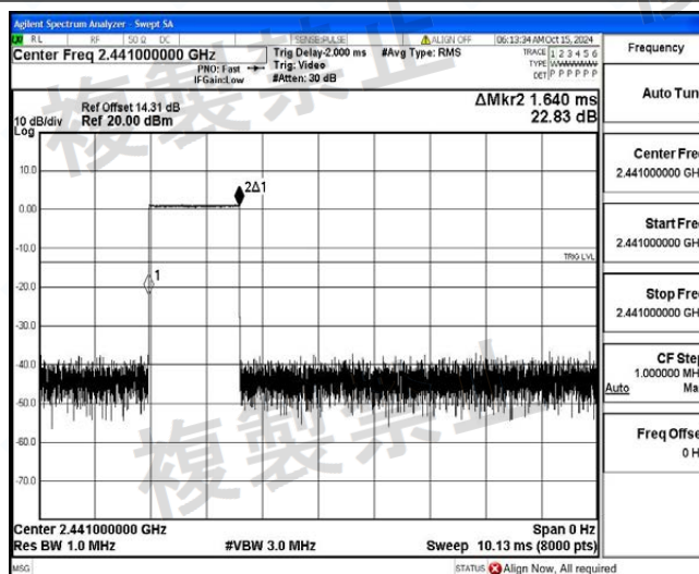
NTNV_DH3_Ant1_Hop
