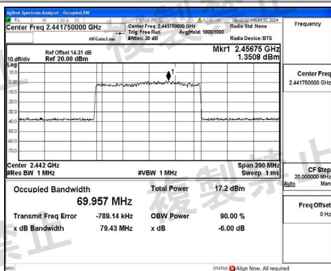
NTLV_DH5_Ant1_Hop
