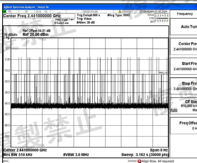
NTLV_3DH3_Ant1_Hop
