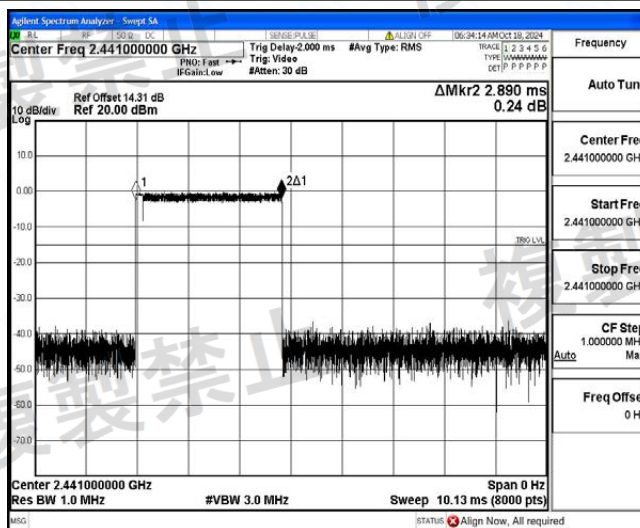
NTLV_2DH5_Ant1_Hop
