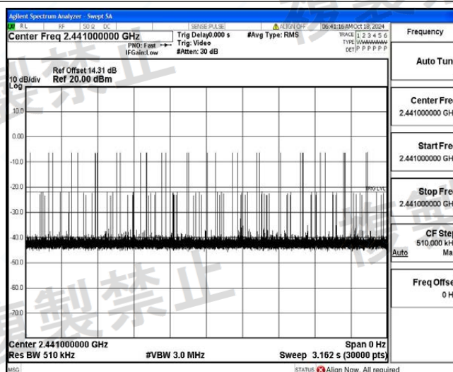
NTLV_2DH3_Ant1_Hop
