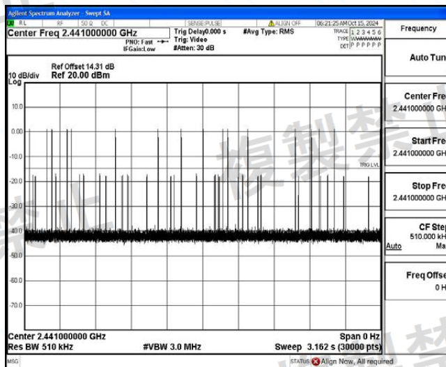
NTNV_2DH5_Ant1_Hop
