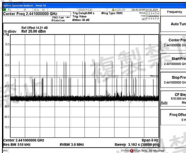
NTHV_2DH5_Ant1_Hop
