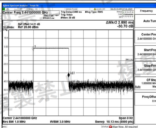
NTLV_DH5_Ant1_Hop
