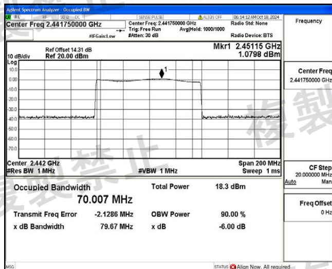
NTHV_2DH5_Ant1_Hop
