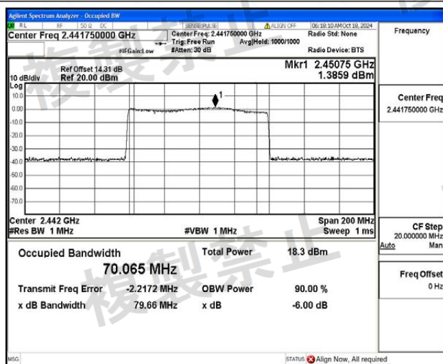
NTLV_3DH5_Ant1_Hop
