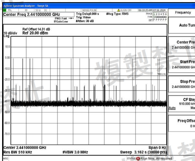
NTHV_DH5_Ant1_Hop
