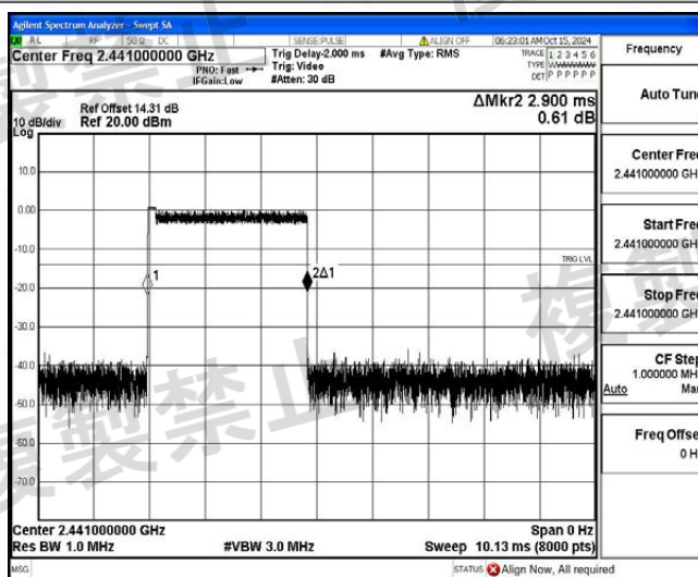
NTNV_3DH5_Ant1_Hop
