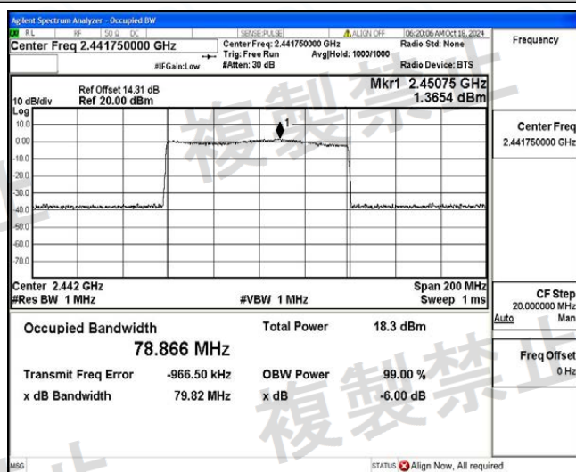
NTHV_3DH5_Ant1_Hop
