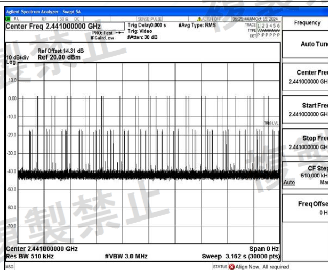
NTNV_3DH3_Ant1_Hop
