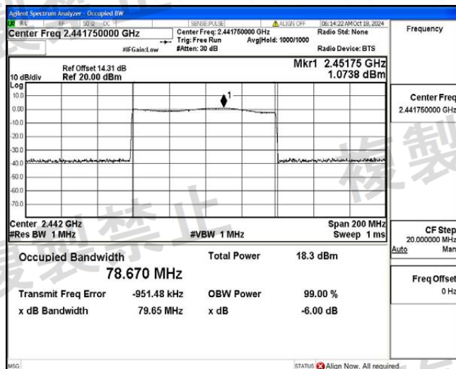
NTLV_2DH5_Ant1_Hop
