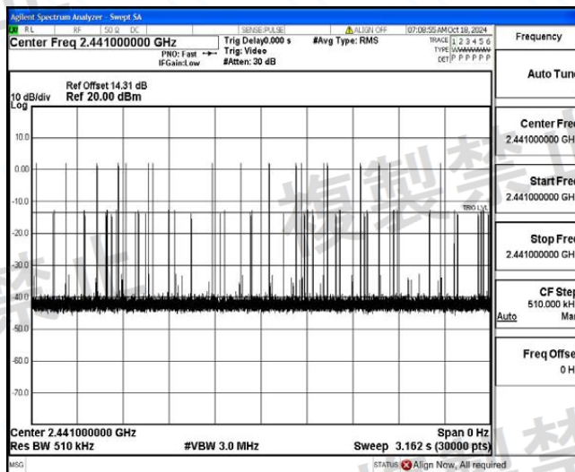
NTHV_3DH5_Ant1_Hop
