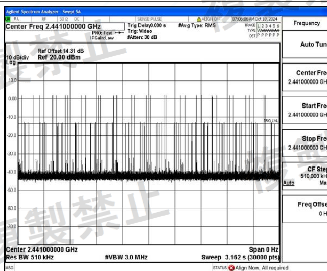
NTHV_3DH3_Ant1_Hop
