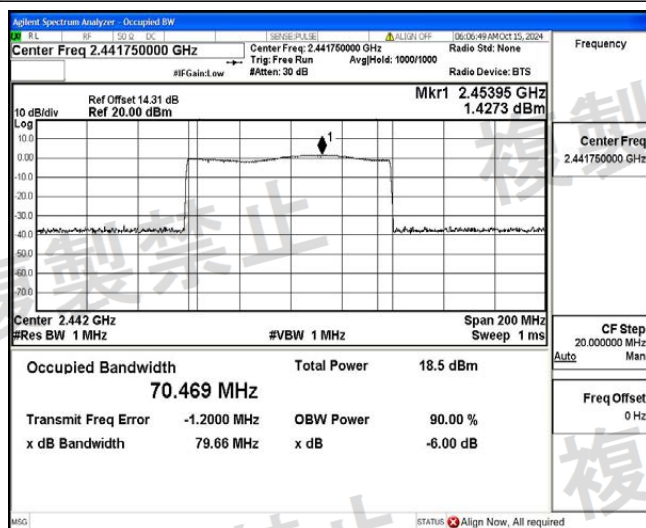
NTNV_2DH5_Ant1_Hop
