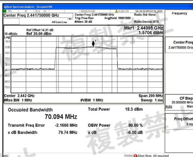
NTHV_DH5_Ant1_Hop
