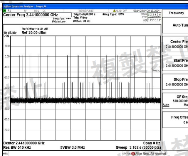
NTNV_DH5_Ant1_Hop
