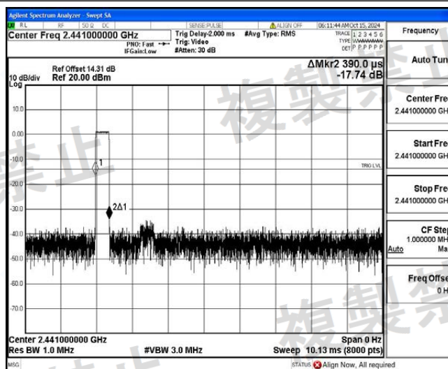
NTNV_DH1_Ant1_Hop
