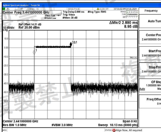
NTLV_3DH5_Ant1_Hop
