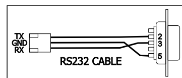
Σχήμα 2: Καλώδιο RS232
