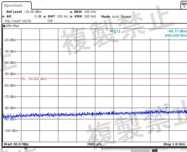
NTNV-11G-Ant1-2412-30~1000-PASS
