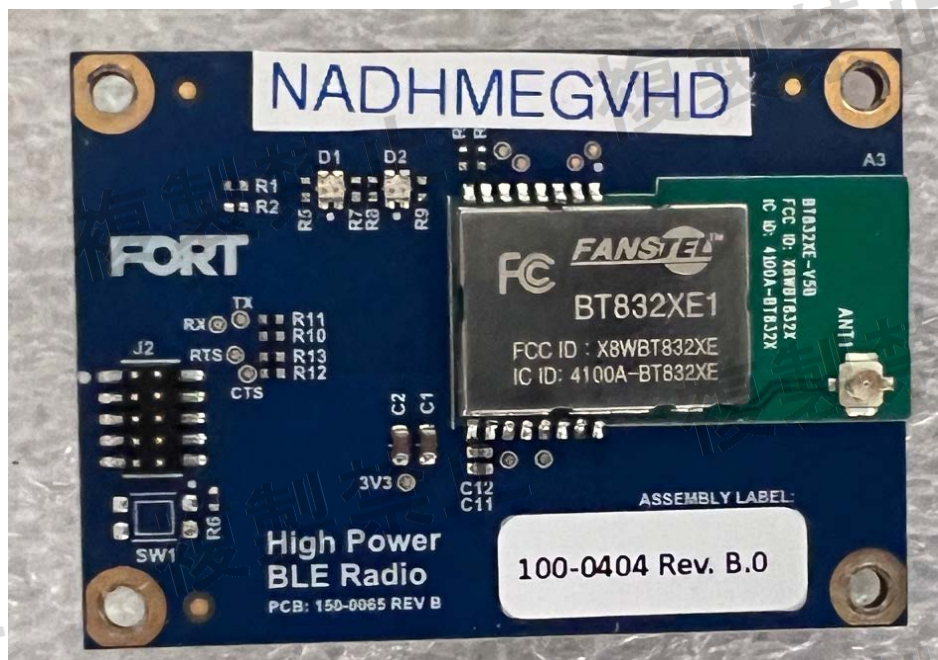
Fig. 7 BLE PCB Primary Side View
