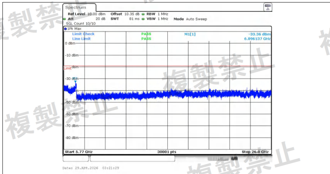
NTNV_11AC80SISO_Ant1_5210_30~5123.2
