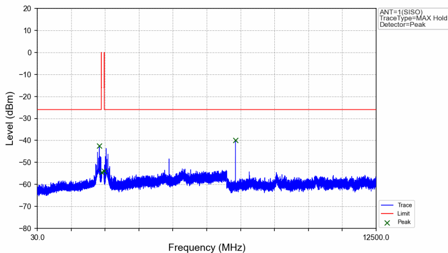
1M_2440MHz_Ant1_NTNV
