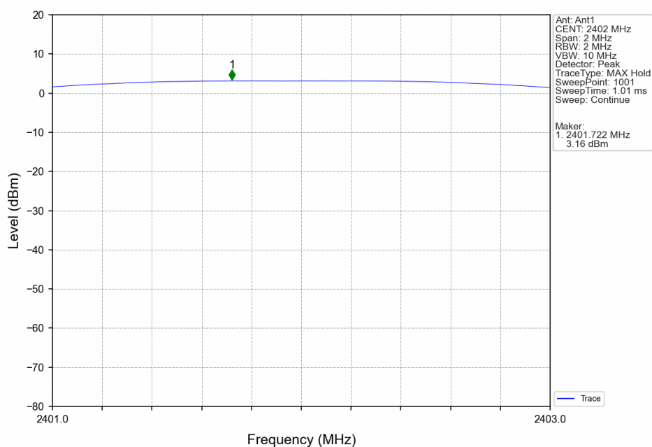
1M_2402MHz_Ant1_NTNV
