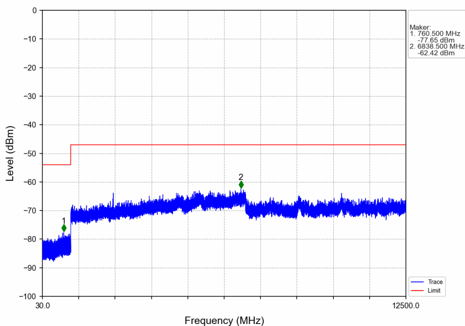
1M_2480MHz_Ant1_NTNV
