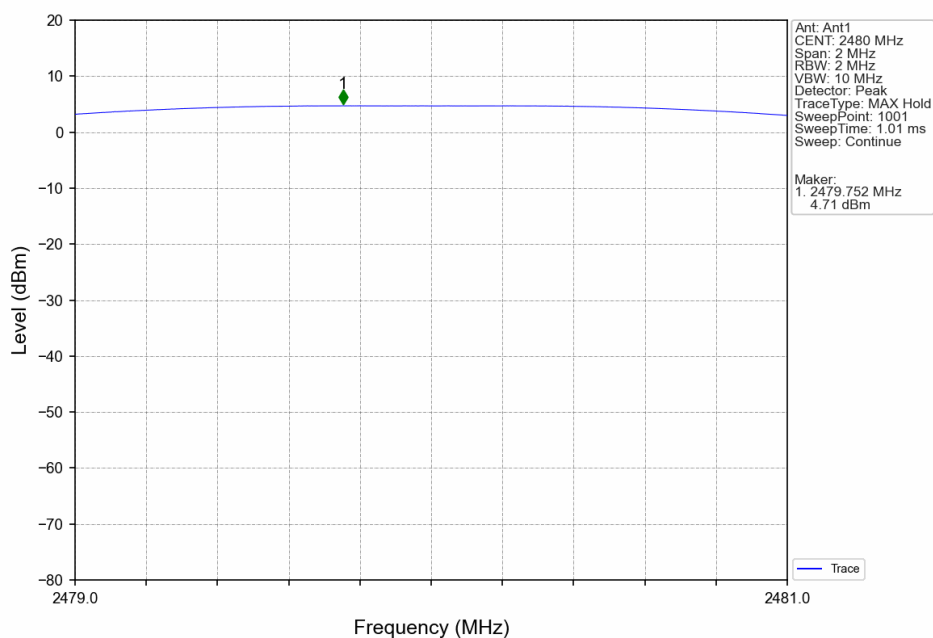
1M_2480MHz_Ant1_NTNV
