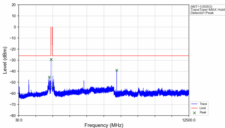
1M_2402MHz_Ant1_NTNV
