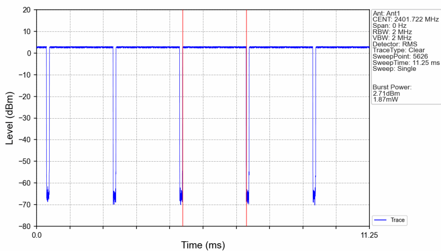
1M_2402MHz_Ant1_NTNV
