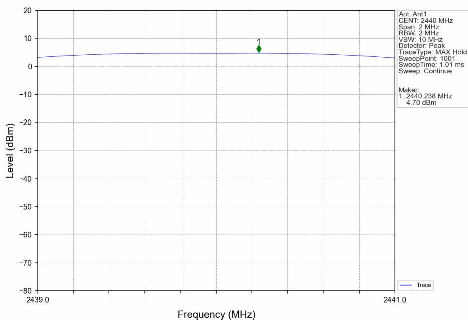
1M_2440MHz_Ant1_NTNV
