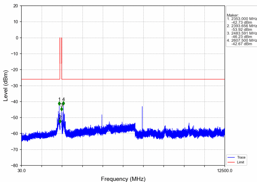
1M_2480MHz_Ant1_NTNV
