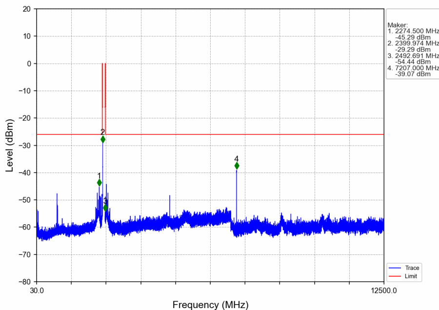
1M_2402MHz_Ant1_NTNV
