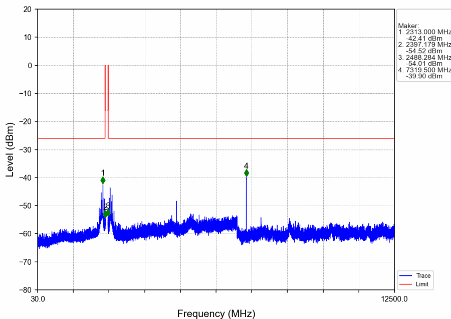
1M_2440MHz_Ant1_NTNV
