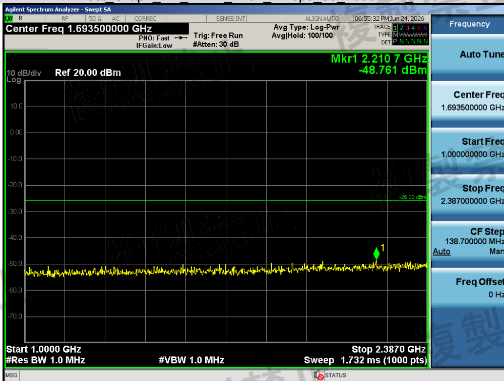
Test_Graph_BR_ANT1_2402_1Mbps_1000_2387MHz_HV
