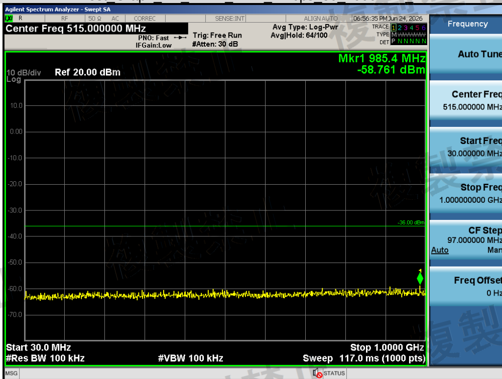
Test_Graph_BR_ANT1_2441_1Mbps_30_1000MHz_NV
