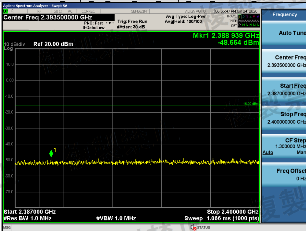
Test_Graph_BR_ANT1_2441_1Mbps_2387_2400MHz_NV
