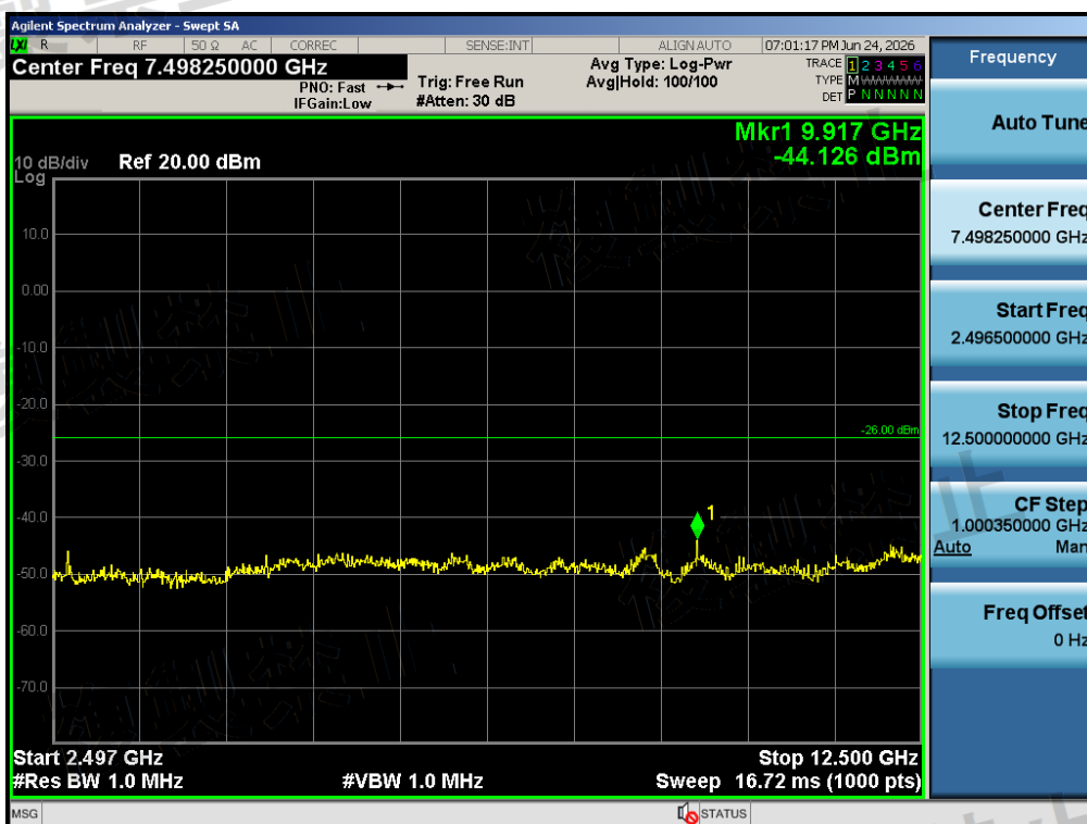
Test Graph BR ANT1 2480 1Mbps 2496.5 12500MHz HV
