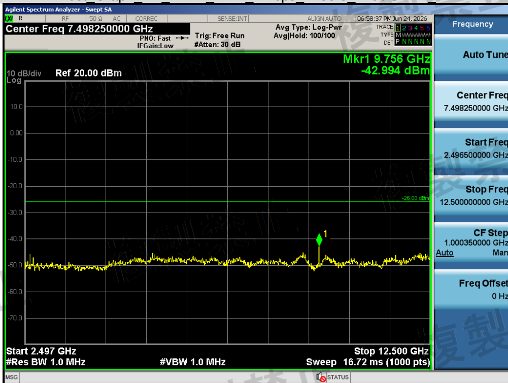
Test_Graph_BR_ANT1_2441_1Mbps_2496.5_12500MHz_HV
