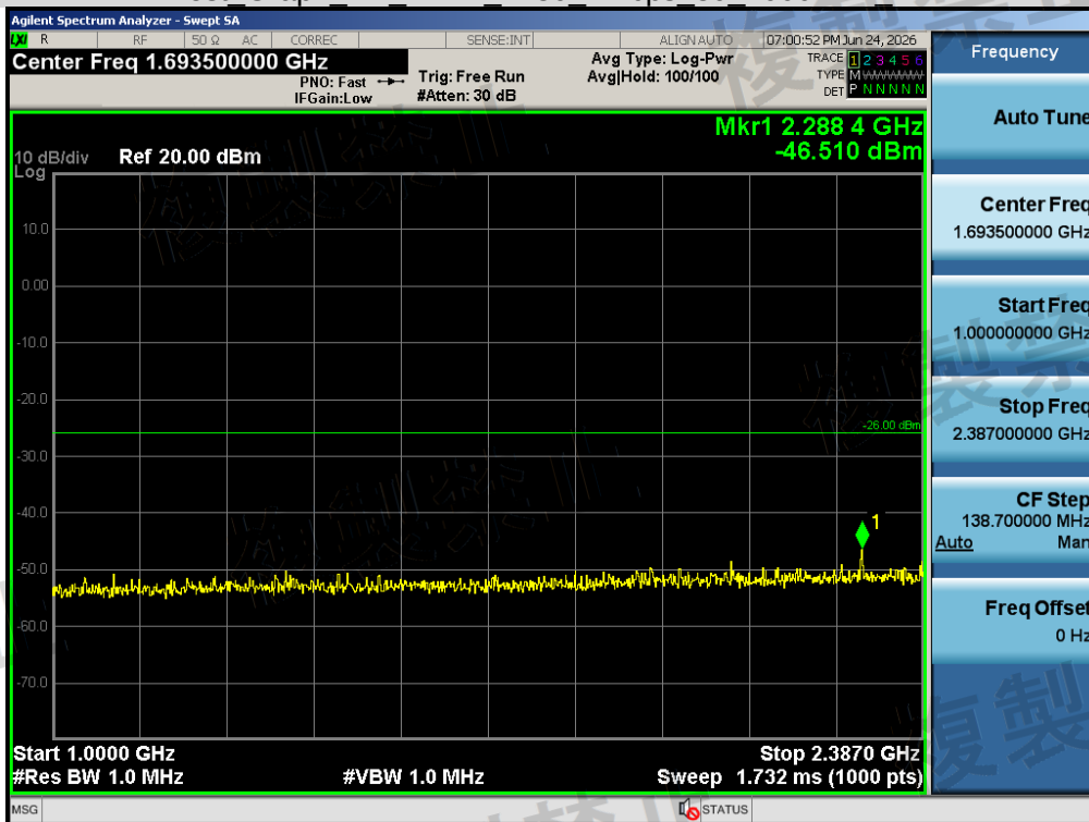
Test_Graph_BR_ANT1_2480_1Mbps_1000_2387MHz_HV
