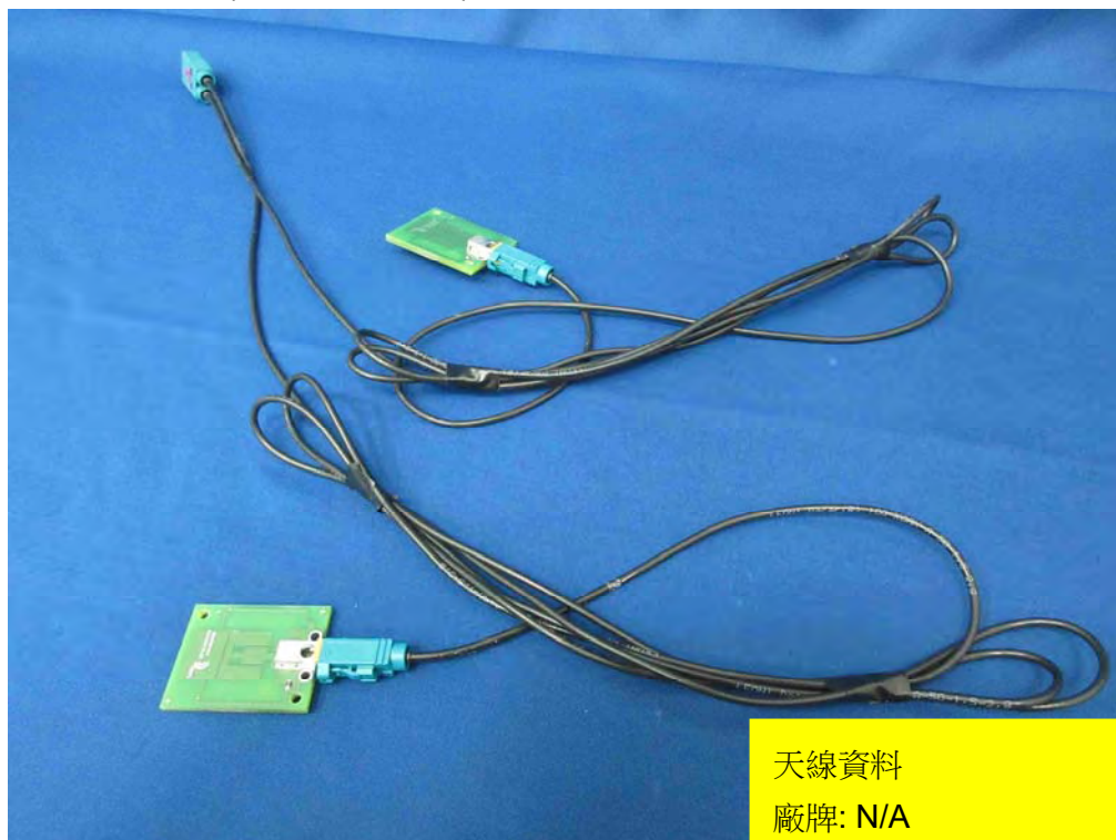
(12) 待測裝置相片 (Port1-2_ANT(2.4G))
