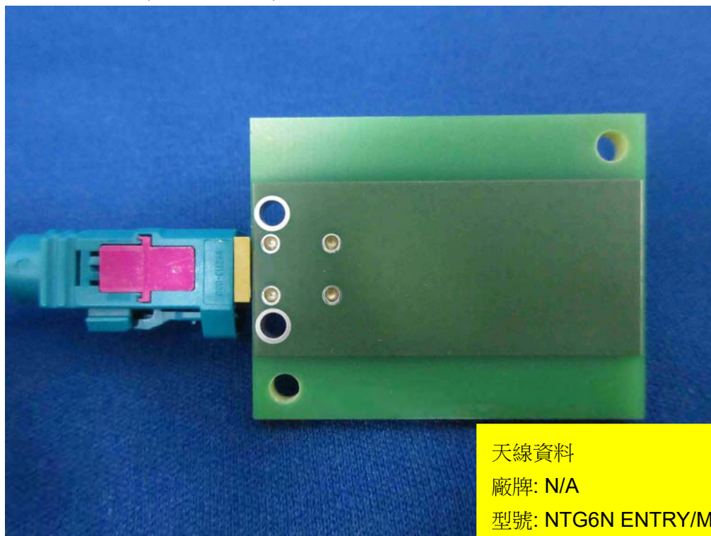
(16) 待測裝置相片 (Port3-1_ANT (5G & BT))
