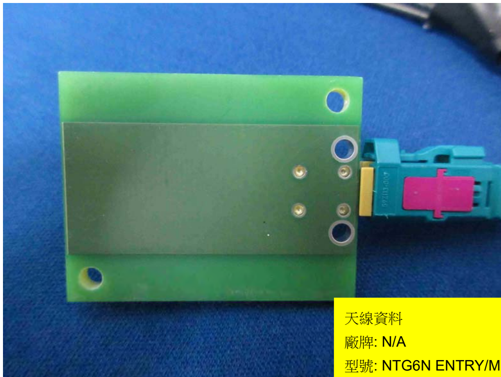
(14) 待測裝置相片 (Port2-4_ANT)
