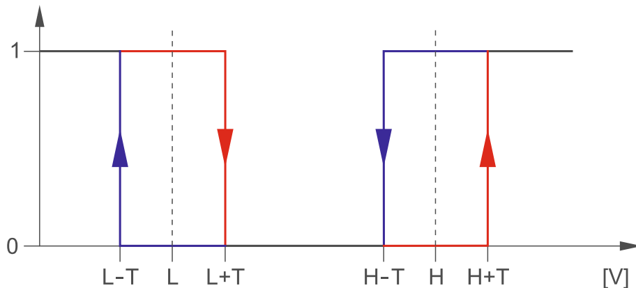
Fig. 20. Mode de fonctionnement de l'entrée analogique. 0 – état normal (pas de violation), 1 – seuil dépassé (violation), L – seuil inférieur, L + T – seuil inférieur plus tolérance, H – seuil supérieur, H + T – seuil supérieur plus tolérance.
